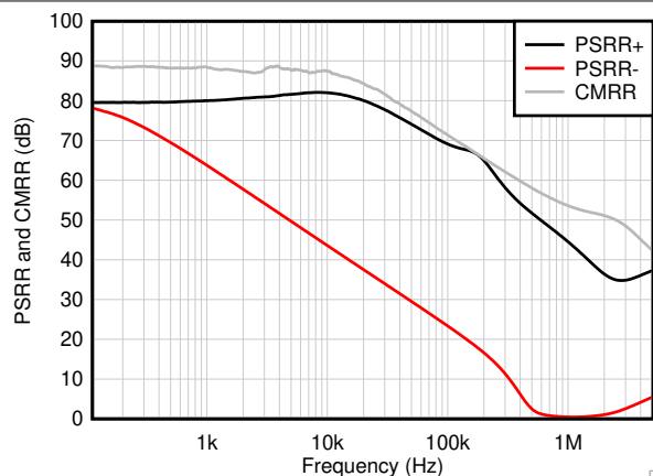
図 7-13. CMRR および PSRR と周波数との関係
