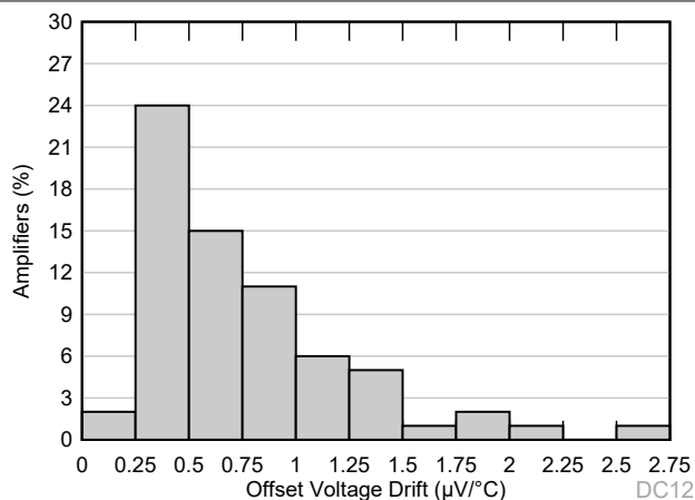
図 7-2. オフセット電圧ドリフトの分布
