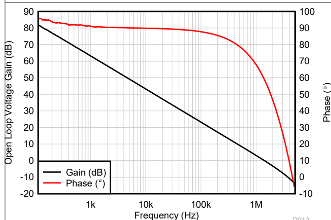
図 7-5. 開ループのゲインおよび位相と周波数との関係
