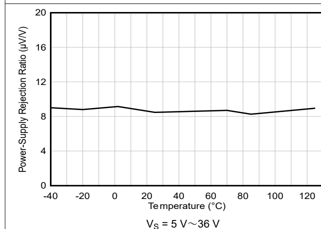
図 6-11. 電源除去比と温度との関係
