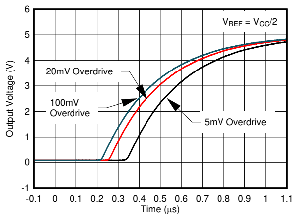
図 5-12. 各種オーバードライブの応答時間、Low から High への遷移
