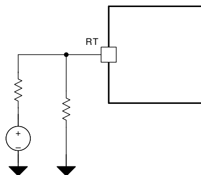
図 8-21. 動的な周波数変更の例
