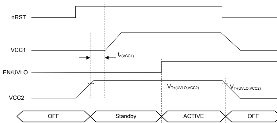
図 8-13. VCC レギュレータのタイミング図
