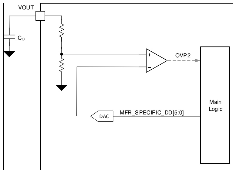
図 8-30. OVP2 の機能ブロック図
