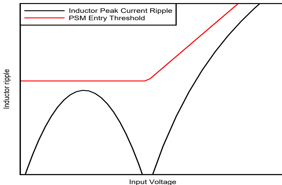
図 8-8. PSM エントリスレッシュホールドおよびリップル電流と入力電圧との関係を示す一般的なグラフ
