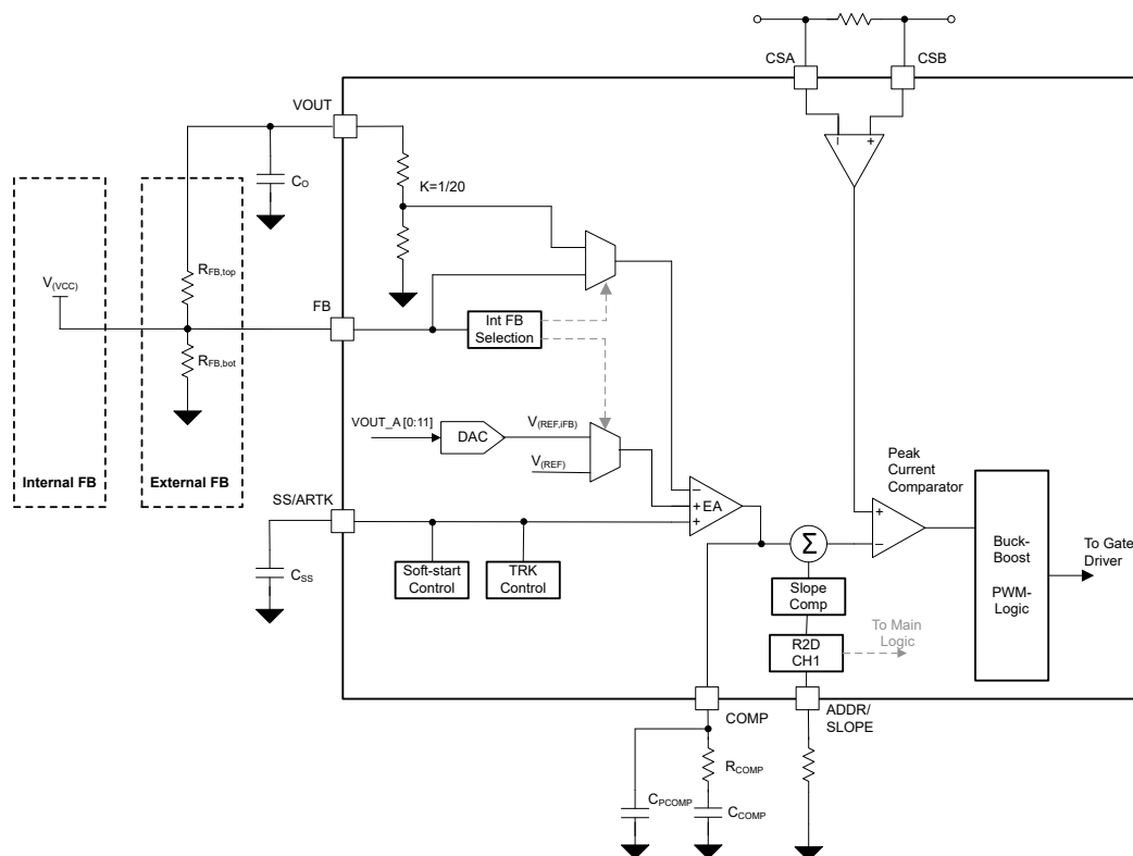
図 8-15. EA 機能ブロック図
