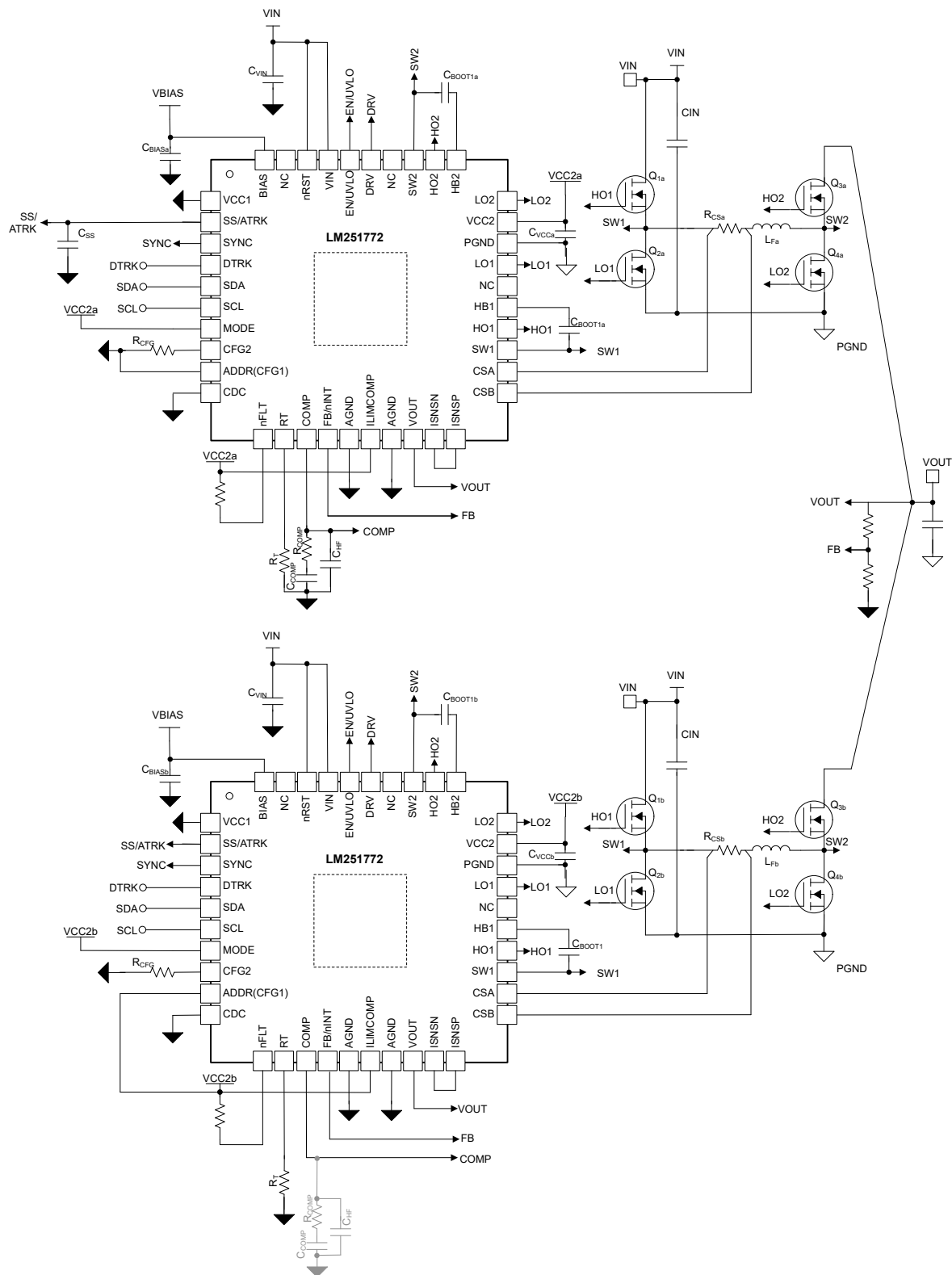
図 10-29. 2 相動作の概略回路図
