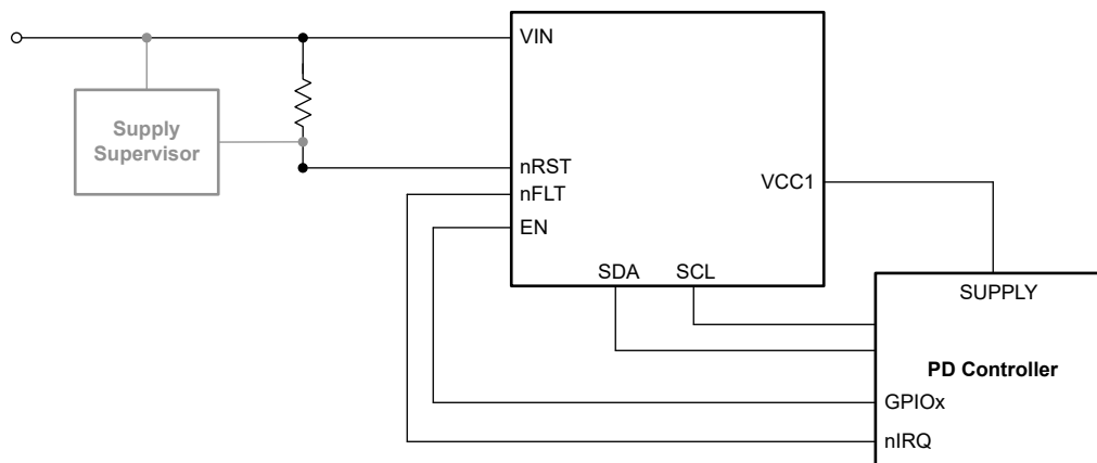
図 8-12. 概略回路図
