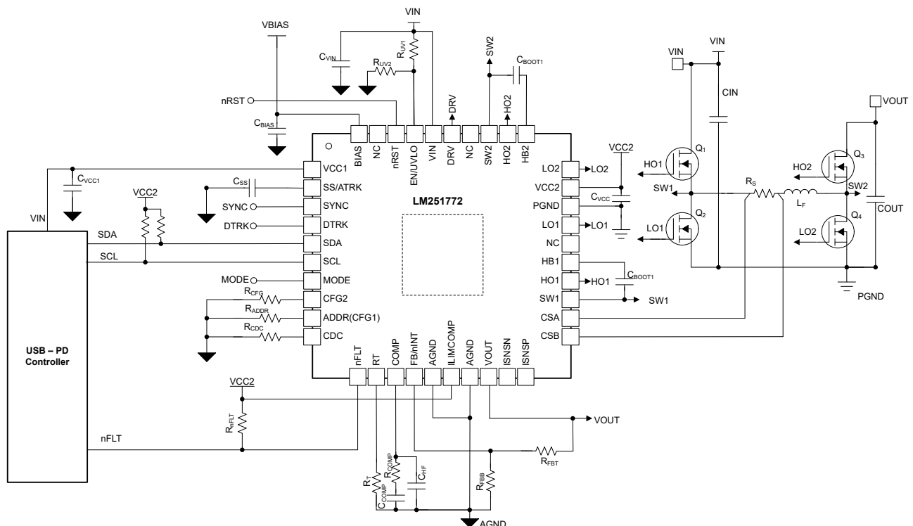
図 10-28. パワーパス付き PD ソースの概略回路図
