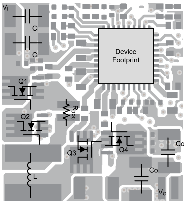
図 10-26. LM34938-Q1 の簡略上層の例
