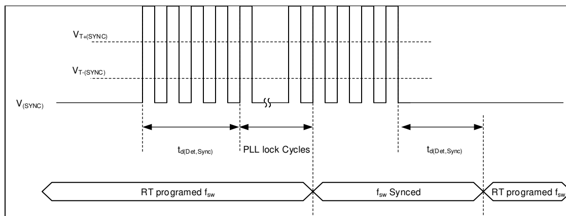
図 8-23. タイミング図の同期機能
