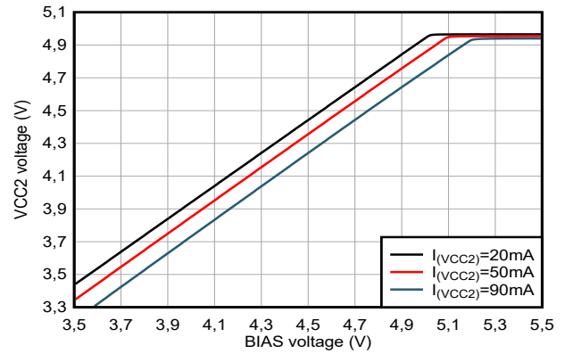
図 6-14. VCC2 LDO 出力電圧と BIAS 電圧との関係 V (VIN) = 2.5V
