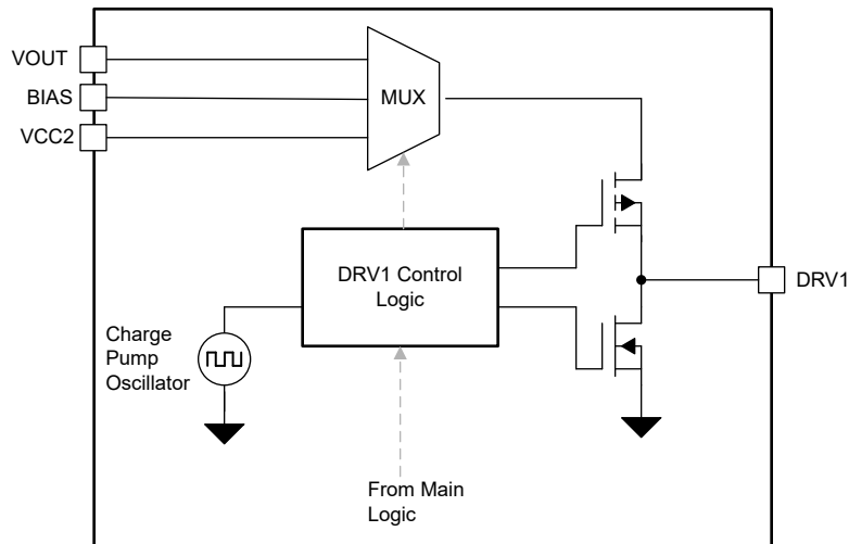
図 8-25. 機能ブロック図 - DRV ピン
