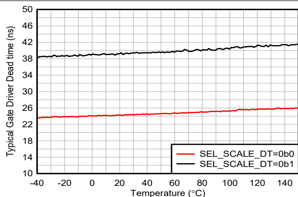
図 6-24. ゲートドライバ遷移 (デッド) 時間とスイッチング周波数との関係 f_{(sw)} = 100\text{kHz} 、SEL_MIN_DEADTIME_GDRV = 0b01、 EN_CONST_TDEAD = 0b0、ローサイド オフ、ハイサイドをオンに します
