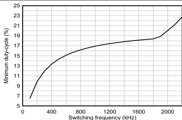
図 6-22. PSM 動作の降圧最小デューティ サイクルとスイッチング周波数との関係 (SYNC_OUT = イネーブル)
