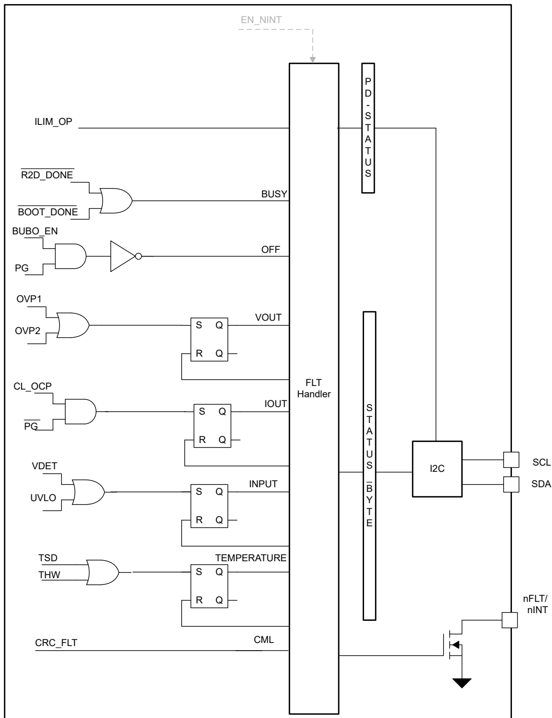
図 8-29. 機能ブロック図フォルト ハンドラ
