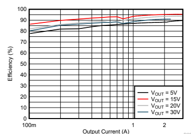
効率と出力電流との関係、 V_i = 12\text{V} 、PSM
