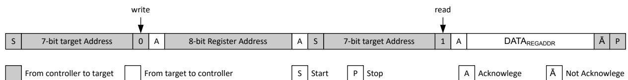
図 8-36. 定義されたレジスタ アドレスからの単一読み取り
