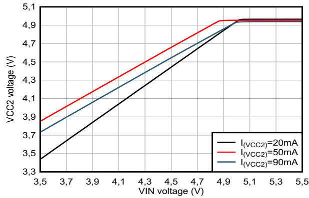
図 6-13. VCC2 LDO 出力電圧と VIN 電圧との関係 V (BIAS) = 0V
