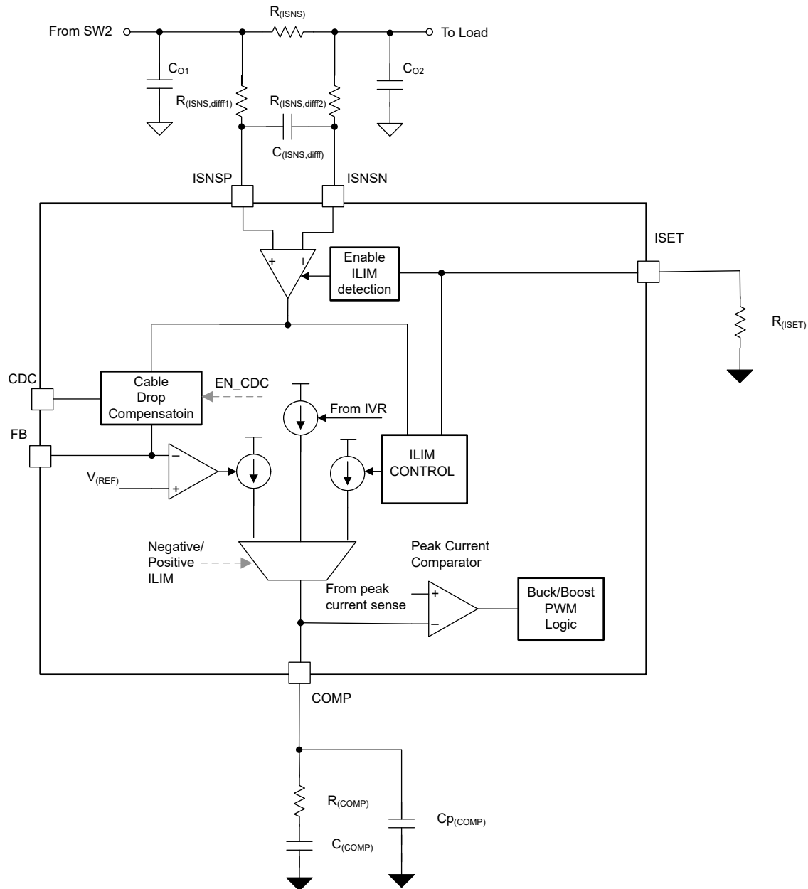
図 8-18. 電流モニタの機能ブロック図
