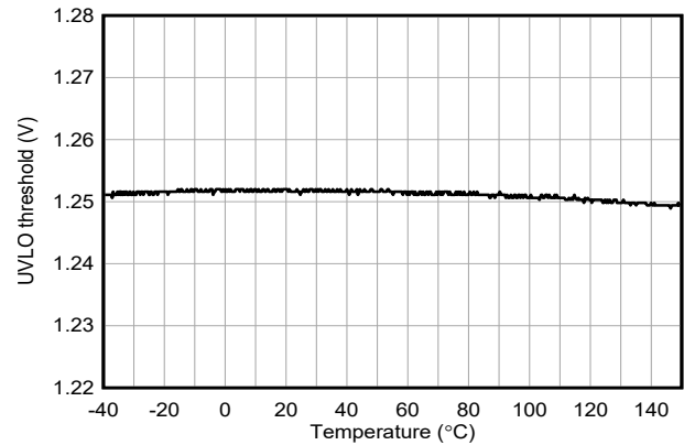
図 6-16. EN/UVLO スレッシュホールドと温度との関係
