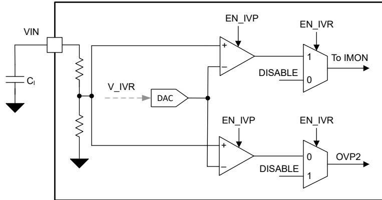
図 8-31. 機能ブロック図 IVP/IVR
