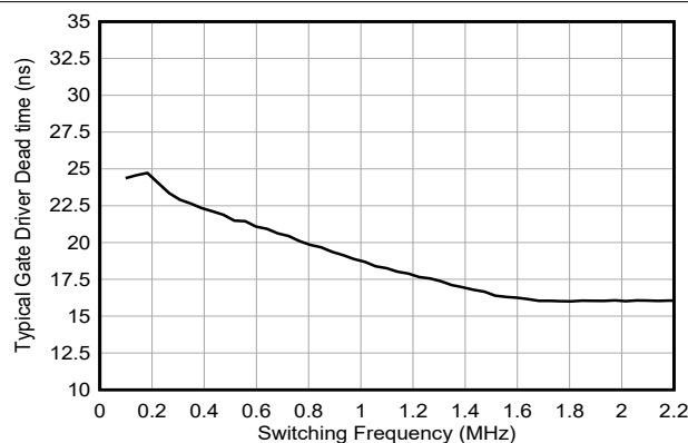
図 6-23. ゲートドライバ遷移 (デッド) 時間とスイッチング周波数との関係 SEL_MIN_DEADTIME_GDRV = 0b01、SEL_SCALE_DT = 0b0、 EN_CONST_TDEAD = 0b0
