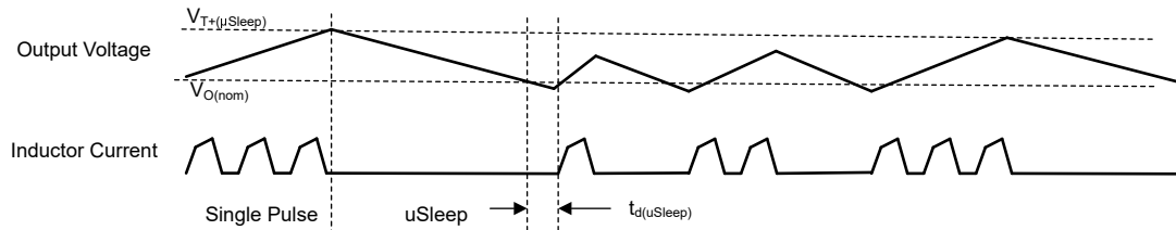
図 8-7. パワーセーブモード (μSleep 有効) のタイミング図
