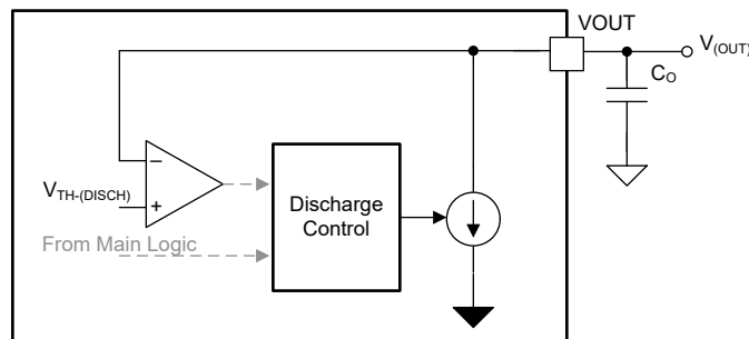
図 8-16. 機能ブロック図出力放電
