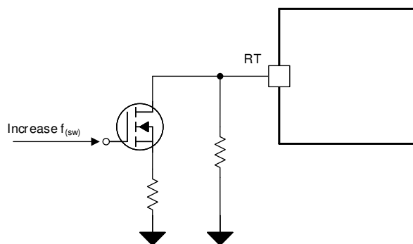
図 8-20. 周波数ホッピングの例
