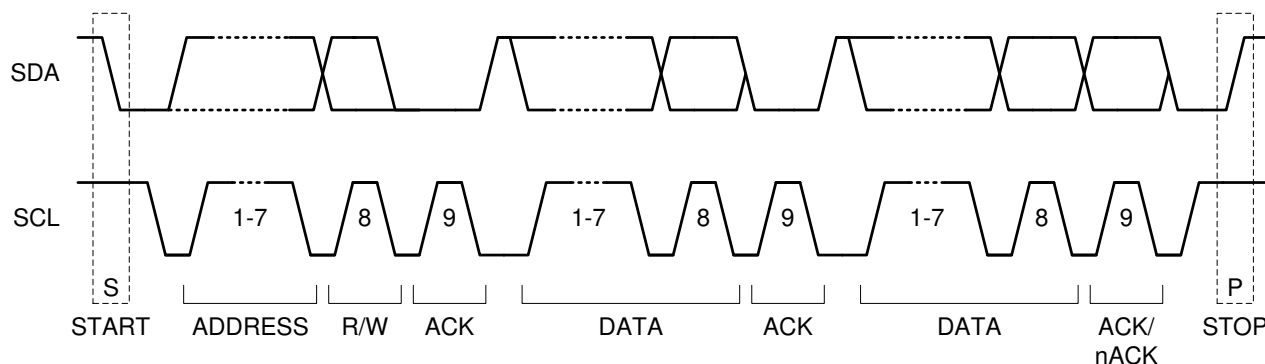
図 8-33. I 2 C スタート/ストップ/アクノリッジのプロトコル
