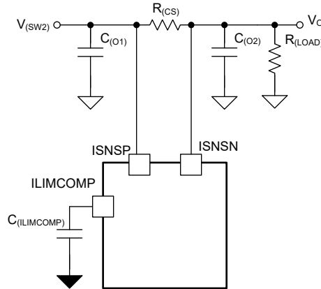
図 8-19. 抵抗性負荷を備えた電流制限部品の概略回路図
