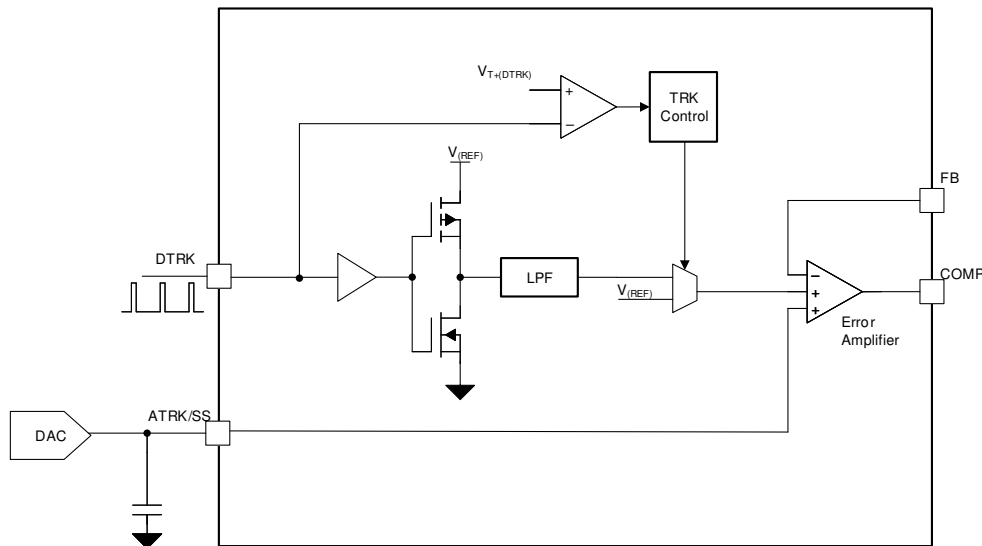
図 8-24. 出力電圧トラッキングの機能ブロック図
