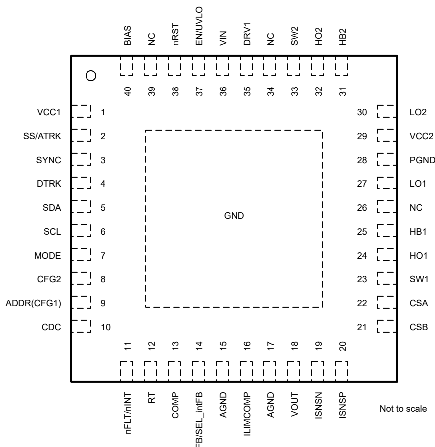
図 5-1. LM34938-Q1 RHA パッケージ、40 ピン QFN (上面図)
