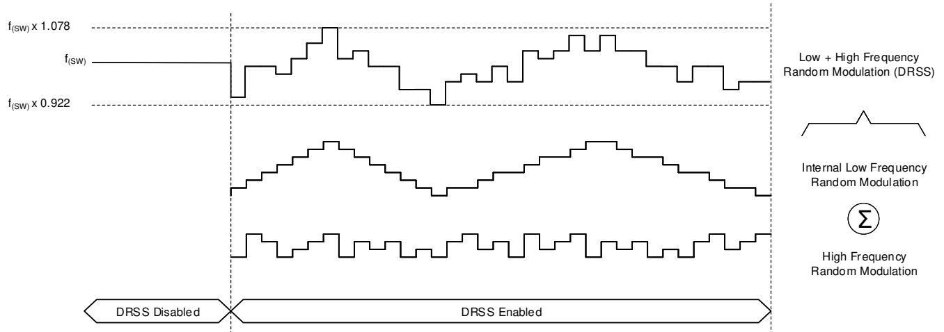
図 8-26. デュアル ランダム スペクトラム拡散
