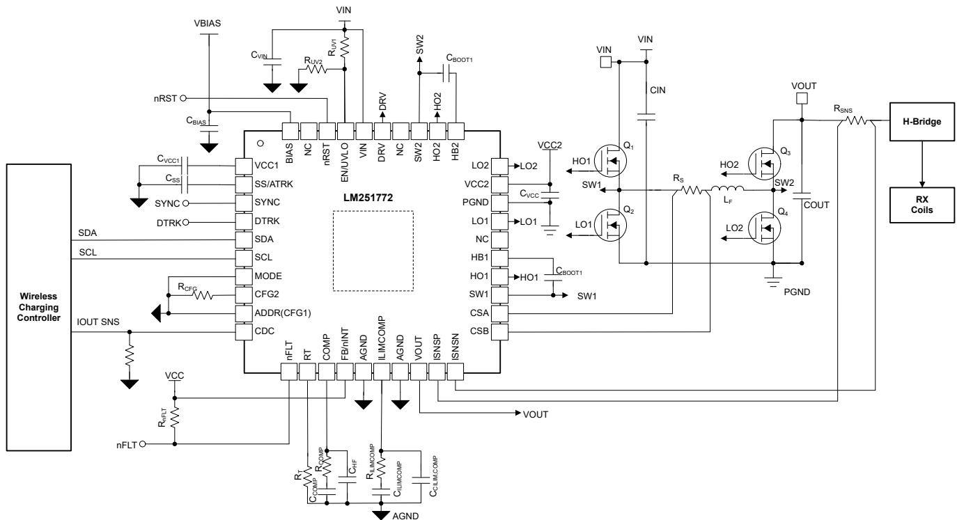
図 10-27. ワイヤレス充電電源の概略回路図
