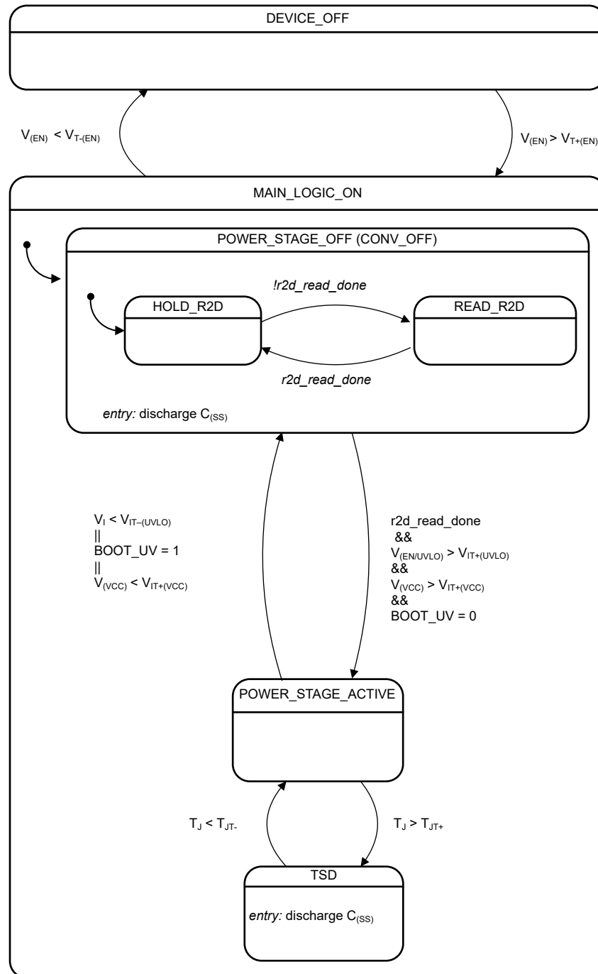
図 8-32. 状態遷移図
