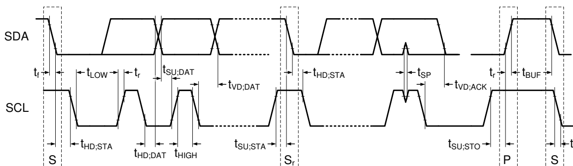
図 8-34. I 2 C データ送信タイミング
