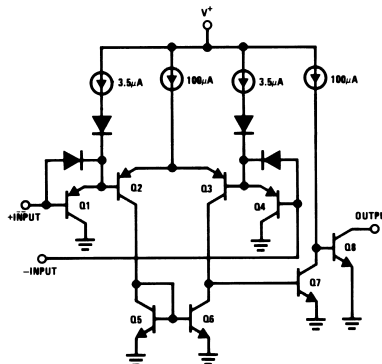
概略回路図
