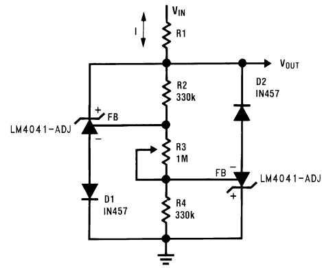
図 8-14. 双方向可変クランプ \pm 2.4V \sim \pm 6V
