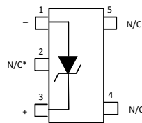
図 4-2. DCK パッケージ 5 ピン SC70 上面図
