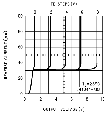
図 8-5. 逆方向特性
