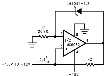
図 8-8. 高精度 1 \mu A ~ 1mA 電流シンク
