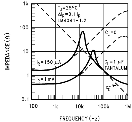
図 5-2. 出カインピーダンス 対 周波数
