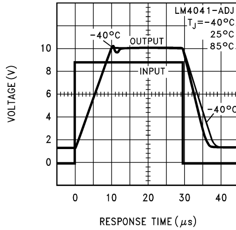
图 5-13. 大信号応答
