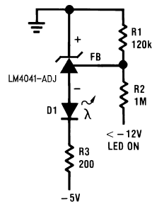
図 8-6. 電圧レベル検出器
