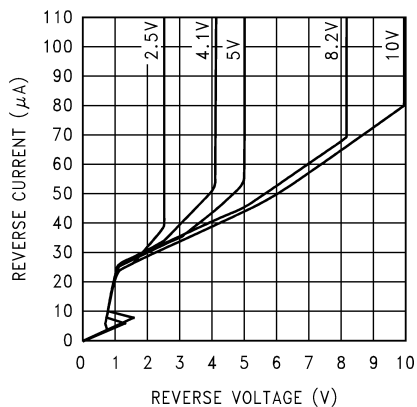
図 5-3. 逆方向特性と最小動作電圧です
