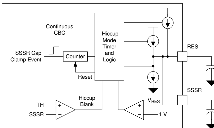
図 7-17. Hiccup Mode Circuitry
