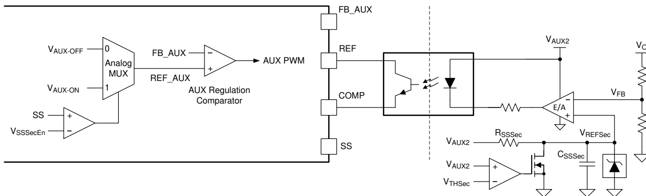
图 7-8. Soft-Start Function
