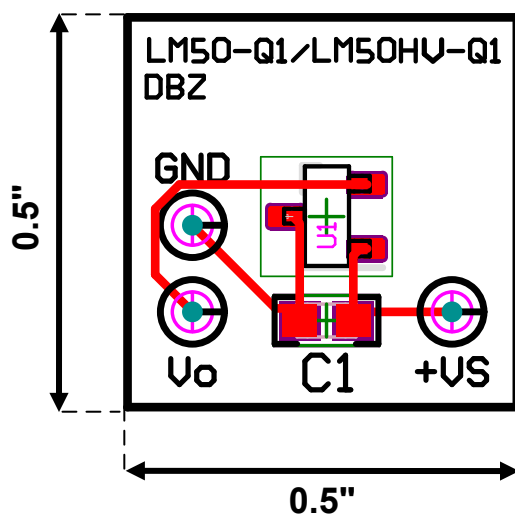
図 8-15. 熱応答曲線の生成に使用するプリント基板 [LM50-Q1 (New Chip および Legacy Chip) と LM50HV-Q1 の新しいテスト設定]
