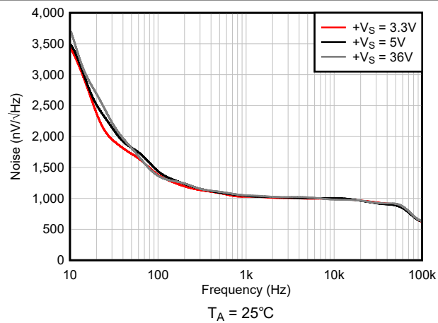
図 6-35. 出力ノイズ密度
