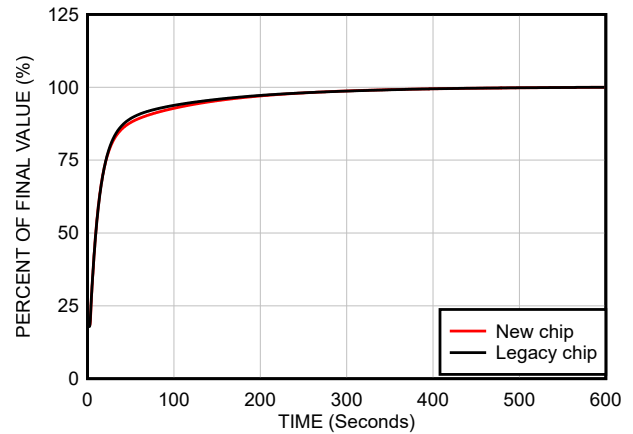
図 6-8. ヒートシンクなしの静止空気中における熱応答 (新しいテスト設定。レガシーチップと新チップの両方)
