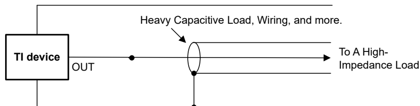
図 8-2. LM50-Q1 および LM50HV-Q1 の容量性負荷にデカップリングは不要
