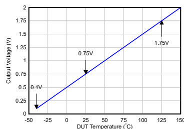
図 3-2. フルレンジ LM50-Q1 ( -40^{\circ}\text{C} \sim 125^{\circ}\text{C} ) および LM50HV-Q1 ( -40^{\circ}\text{C} \sim 150^{\circ}\text{C} )
