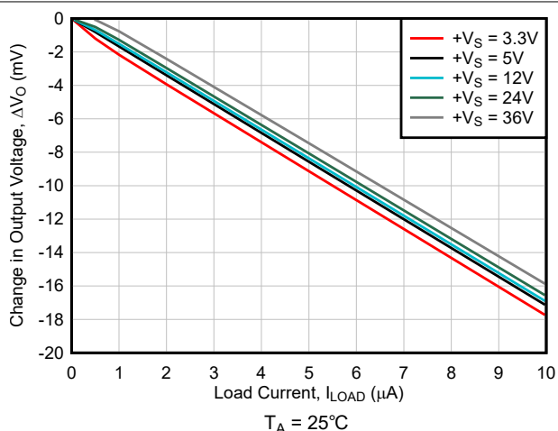
図 6-28. 出力電圧と負荷電流の関係の変化
