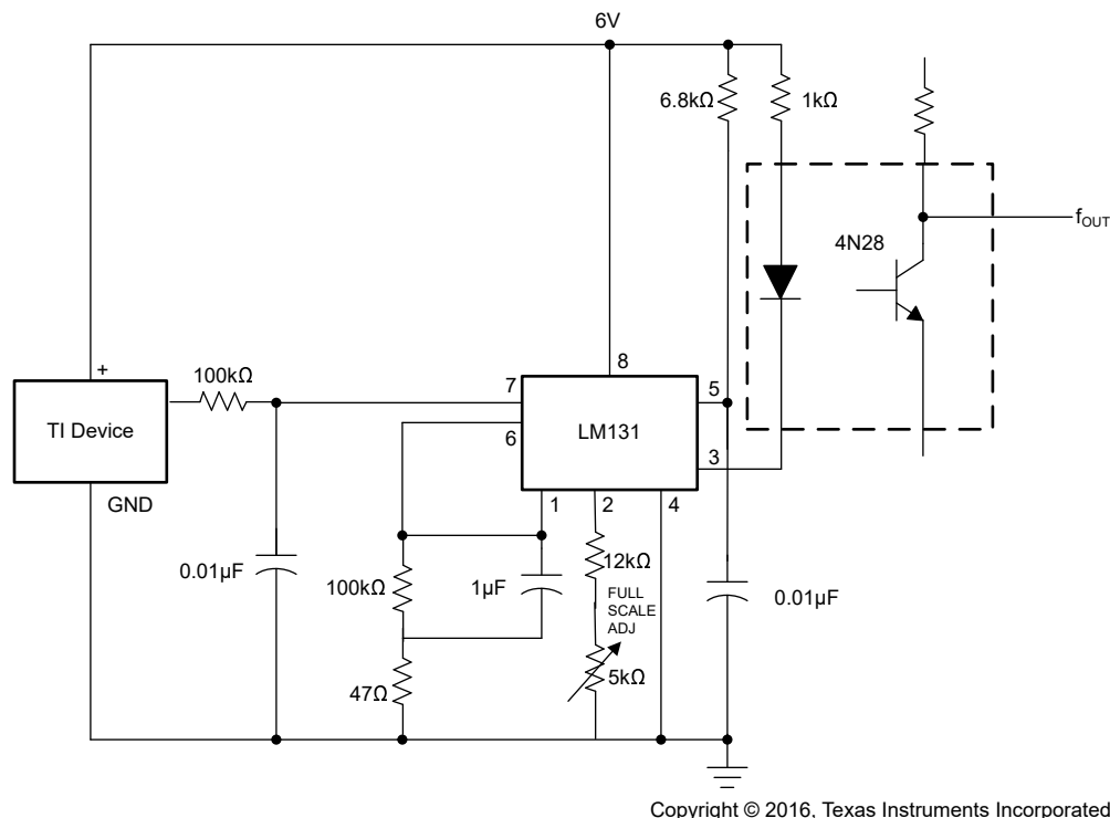
図 8-12. LM50-Q1 および LM50HV-Q1、電圧/周波数コンバータおよび絶縁出力付き
