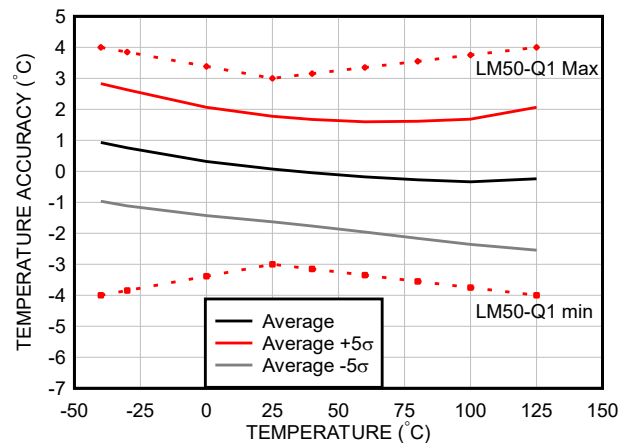
図 6-14. 精度と温度との関係 (新チップ)
