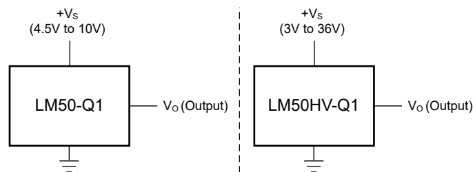
図 8-1. 全範囲の摂氏温度センサ LM50-Q1 (–40°C ~ 125°C) および LM50HV-Q1 (–40°C ~ 150°C)
