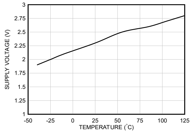
図 6-10. スタートアップ電圧と温度との関係 (新チップ)
