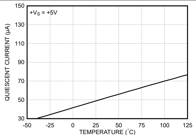
図 6-12. 静止電流と温度との関係 (新チップ)
