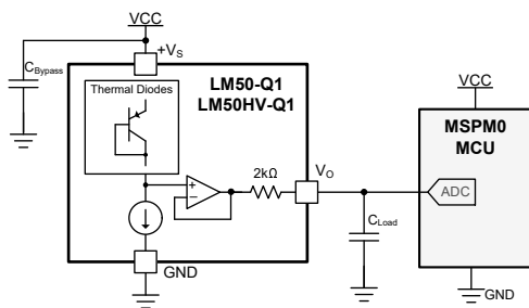
図 3-1. 概略回路図
