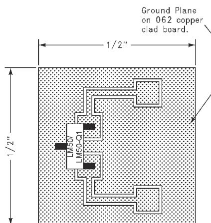
図 8-14. 熱応答曲線生成のヒートシンクに使用するプリント基板 LM50-Q1 (Legacy Chip)
