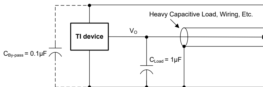
図 8-3. LM50-Q1 および LM50HV-Q1、ノイズ環境用フィルタ付き
