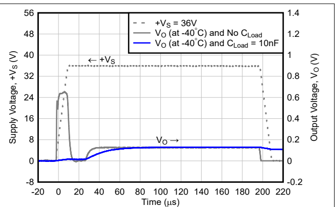
図 8-7. SR = 3.3V/\mu s のときの、 C_{By-pass} なしの +V_S = 36V ステップまでの起動応答 ( C_{Load} および C_{Load} = 10nF )
