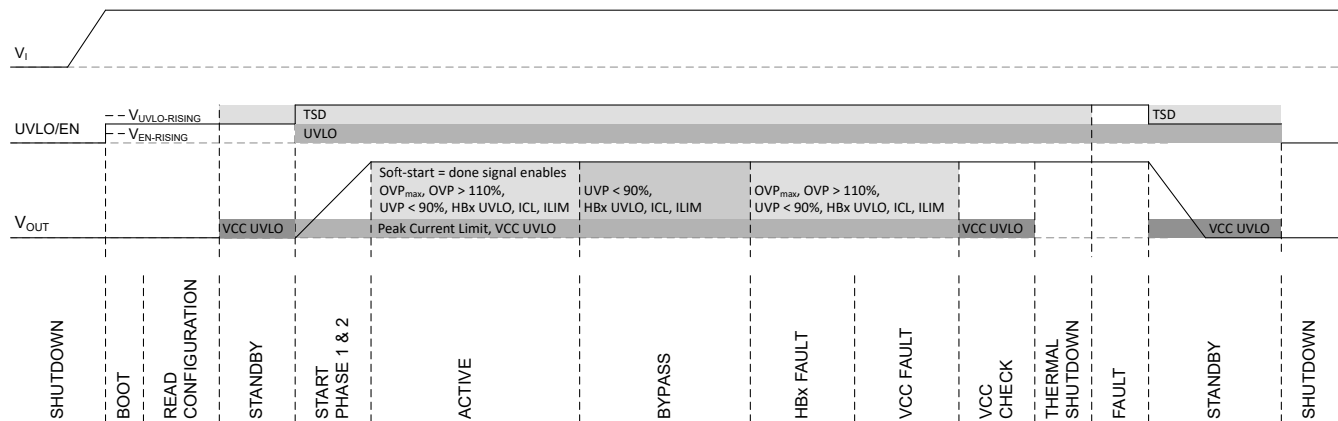
図 6-19. 保護素子
