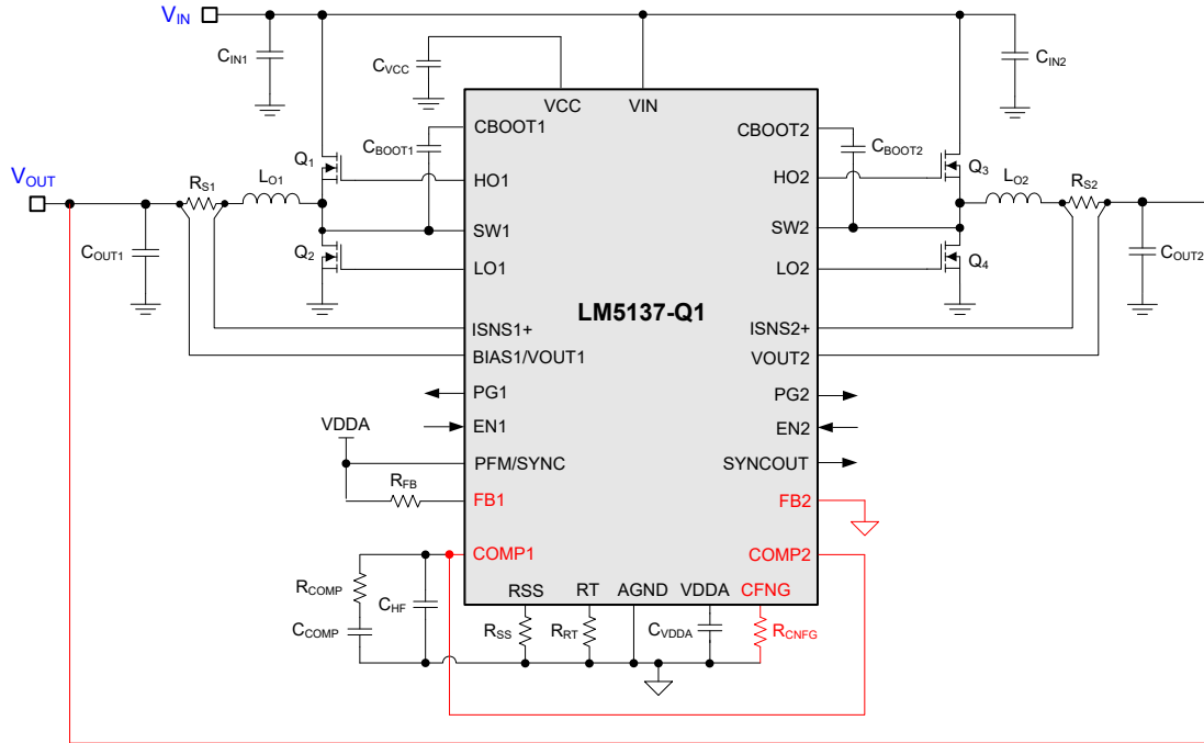
図 7-8. LM5137-Q1 単一出力インターリーブ動作用に構成された 2 相レギュレータの回路図
