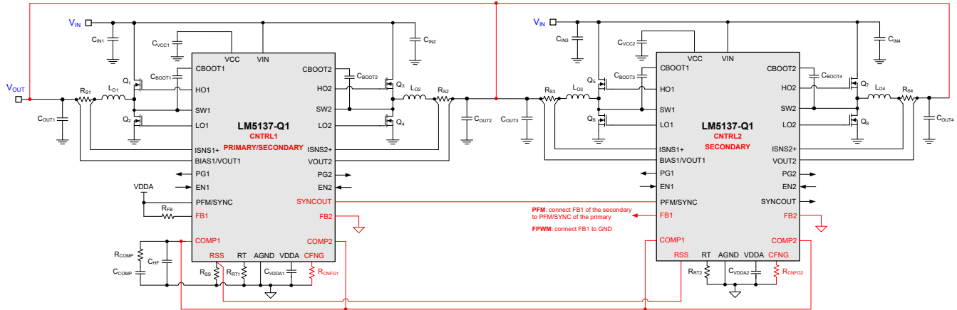
図 7-9. LM5137-Q1 単一出力インターリーブ動作用に構成されたマルチフェーズレギュレータの回路図
