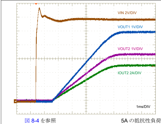
図 6-3. スタートアップ特性
