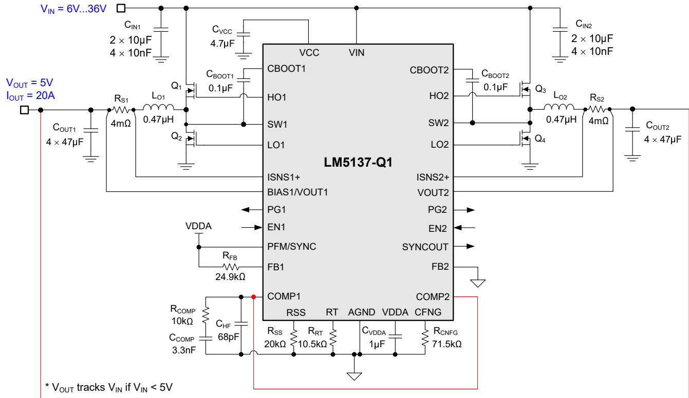
図 8-19. アプリケーション回路 2、LM5137-Q1 2 相降圧レギュレータを 2.1MHz で使用
