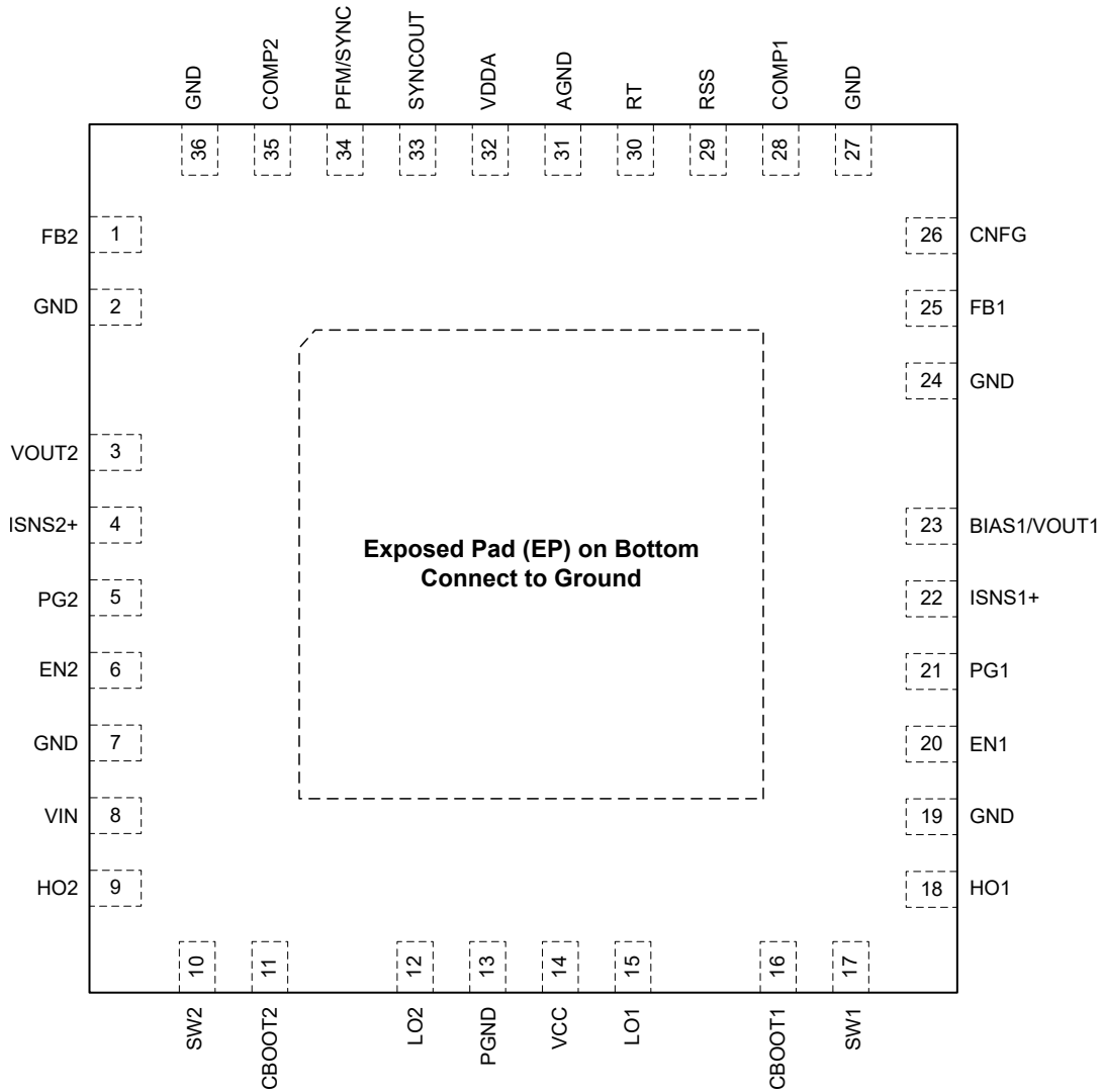
図 5-1. RHA パッケージ、ウェットプル フランク付き 36 ピン VQFN (上面図)
