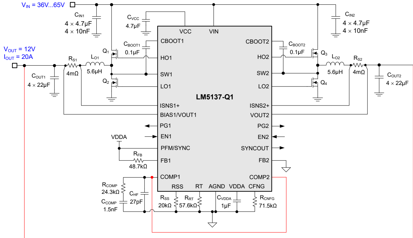
図 8-20. アプリケーション回路 3、LM5137-Q1 2 相降圧レギュレータを 400kHz で使用
