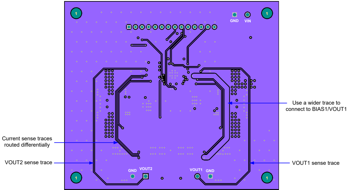
図 8-33. PCB 内層
