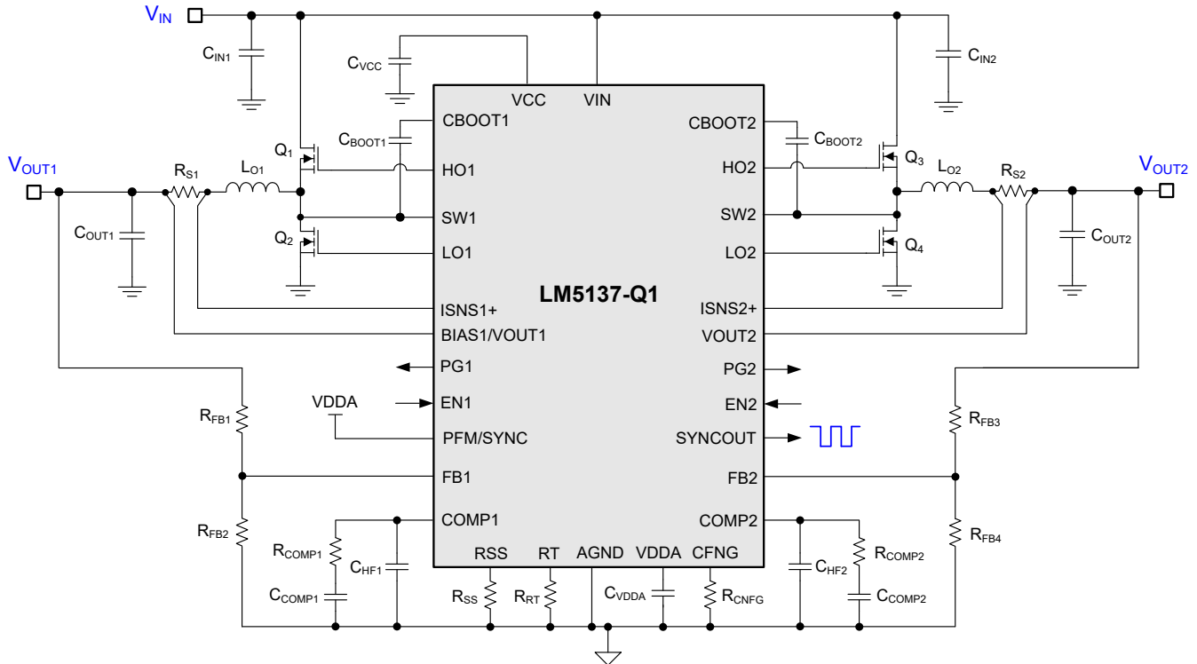
図 7-1. LM5137-Q1 デュアル出力レギュレータの回路図
