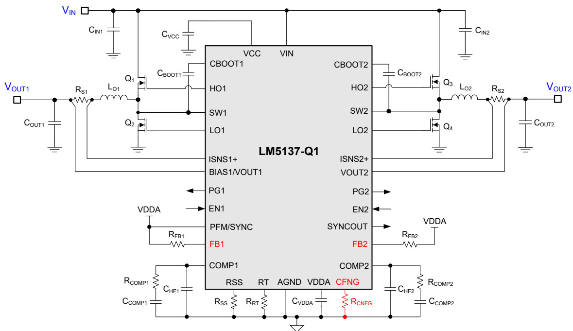
図 7-7. LM5137-Q1 独立したデュアル出力用に構成されたレギュレータの回路図
