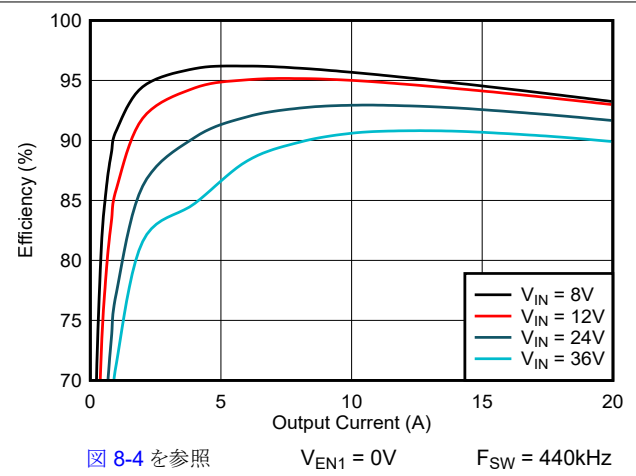
図 6-2. 効率と負荷との関係、3.3V 出力
