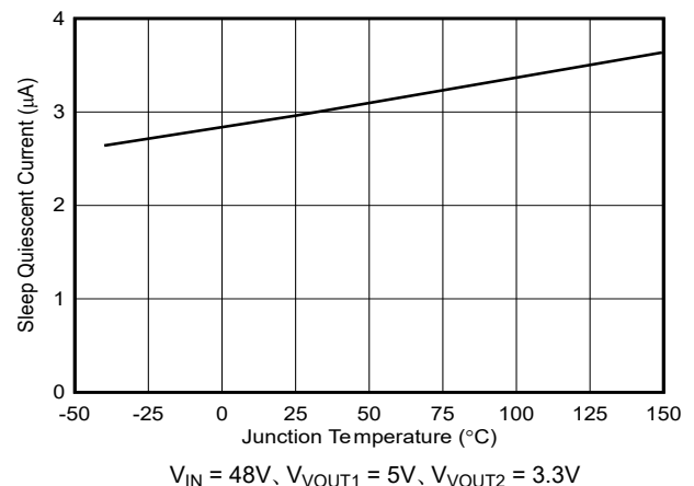
図 6-10. スリープ静止電流と温度との関係
