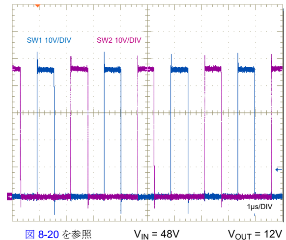
図 6-6. スイッチノード電圧
