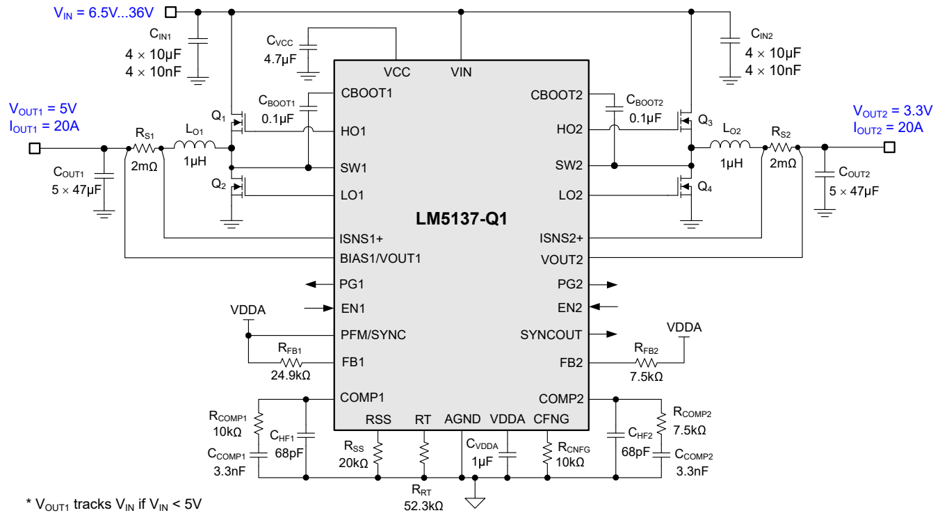
図 8-4. アプリケーション回路 1、LM5137-Q1 降圧レギュレータを 440kHz で使用
