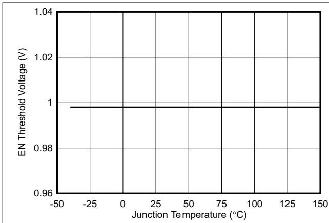
図 6-23. EN 立ち上がりスレッシュヨルド電圧と温度との関係
