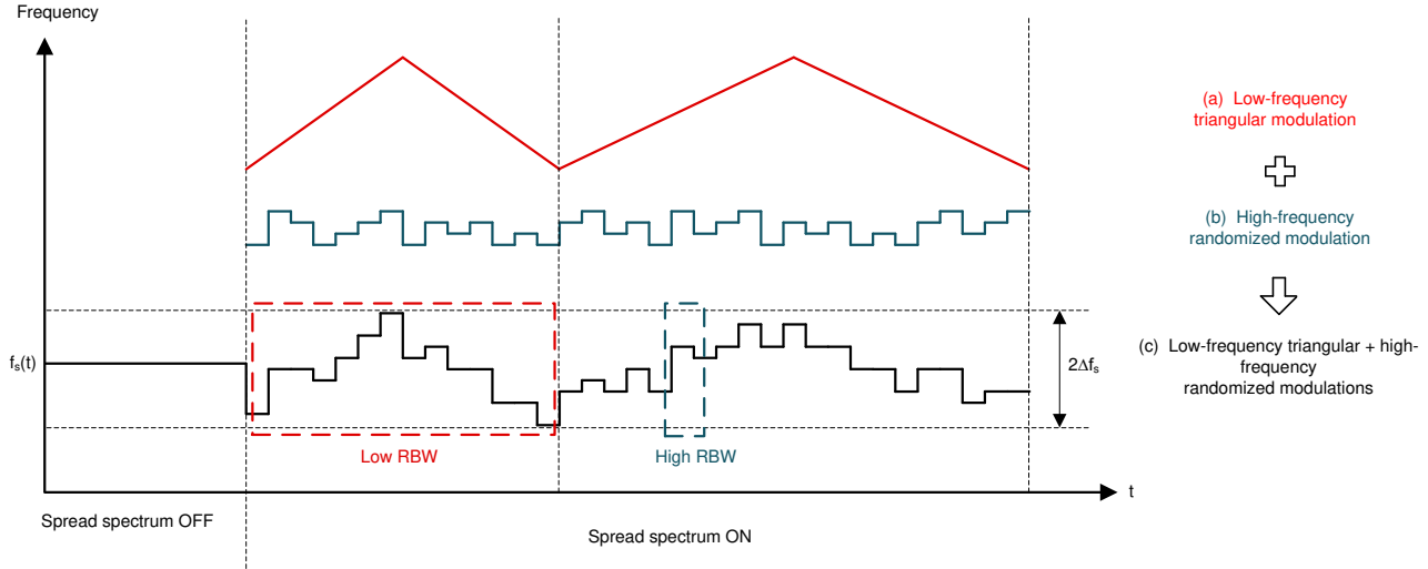
図 7-3. DRSS の実装
