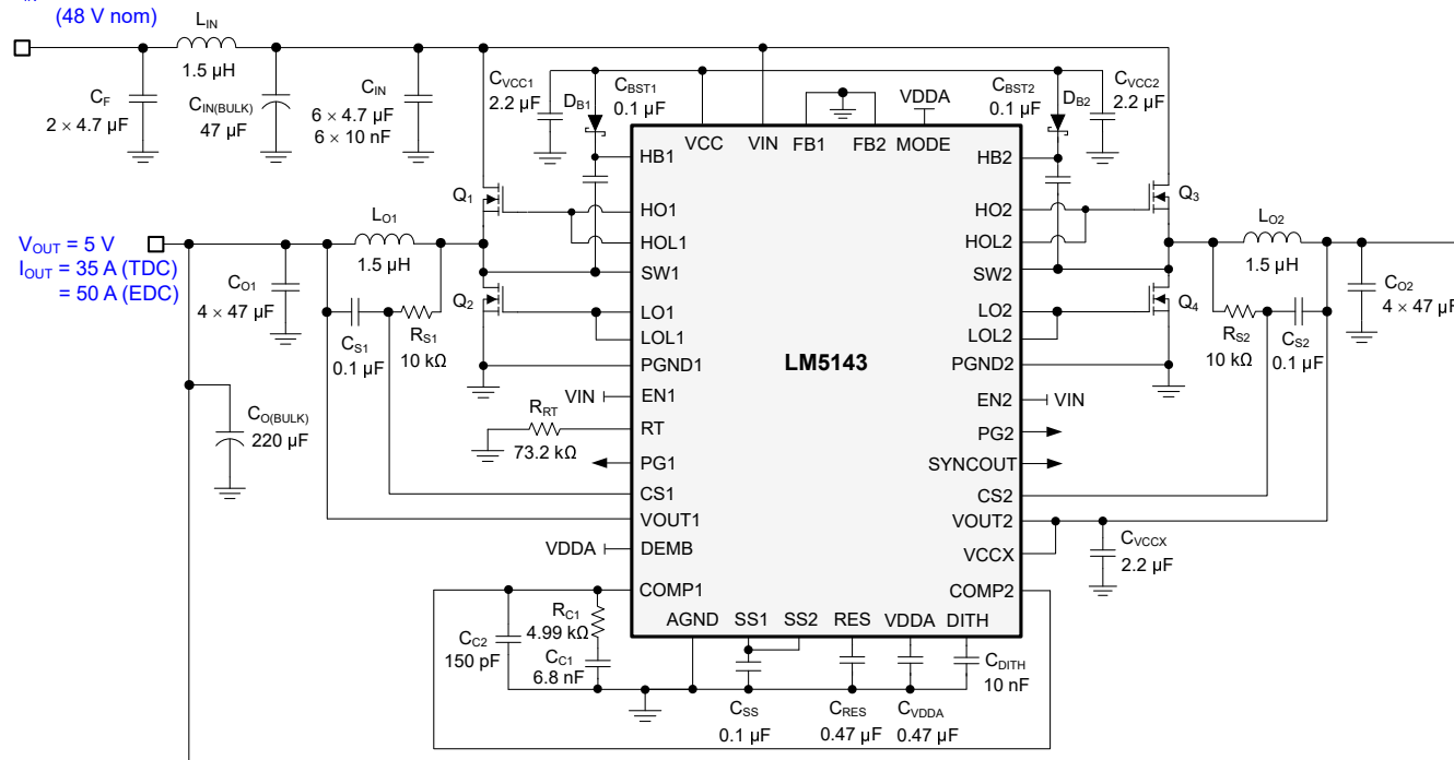
図 10-24. アプリケーション回路 3、LM5143 2 相降圧レギュレータを 300kHz で使用
