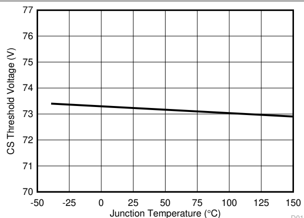
図 8-22. 電流センス (CS1) スレッシュホルドと温度との関係
