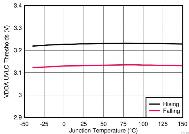
図 8-19. VDDA UVLO スレッシュホルドと温度との関係
