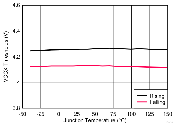
図 8-20. VCCX のオン / オフ・スレッシュホルドと温度との関係
