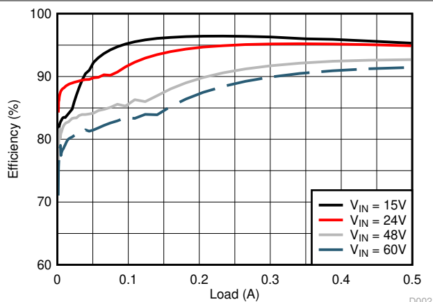
図 5-2. Conversion Efficiency (Linear Scale)
