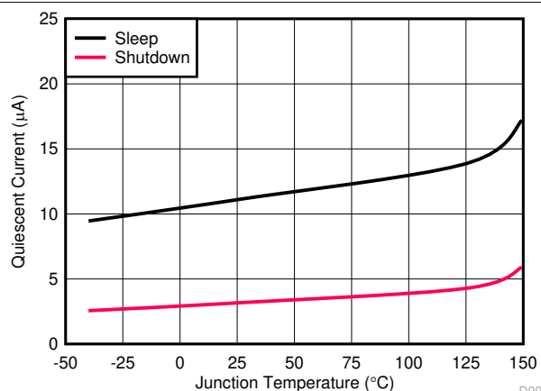
図 5-3. V_{IN} シャットダウンおよびスリープ時の電源電流と温度との関係
