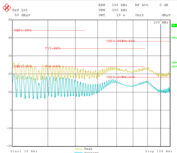
図 7-15. 全負荷スイッチング
