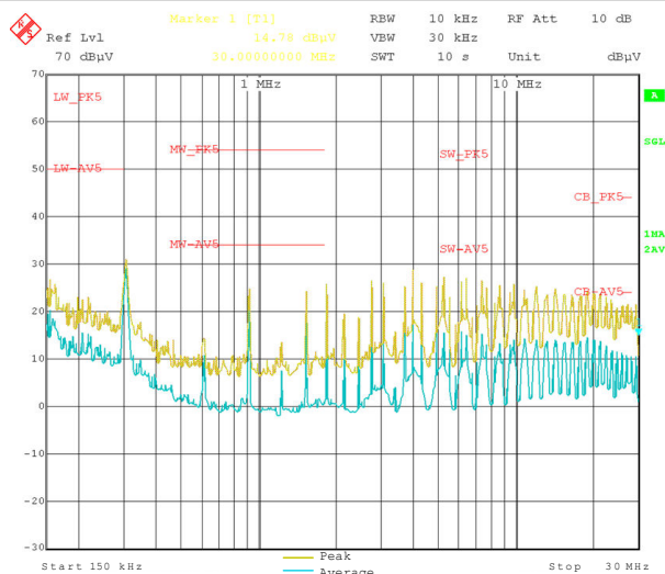
図 7-14. 無負荷スイッチング
