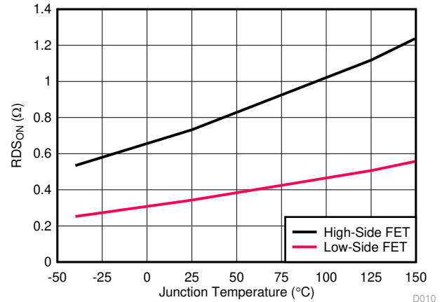
図 5-8. MOSFET のオン状態抵抗と温度との関係
