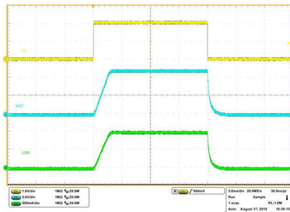
図 7-9. 全負荷時の EN/UVLO による起動とシャットダウン
