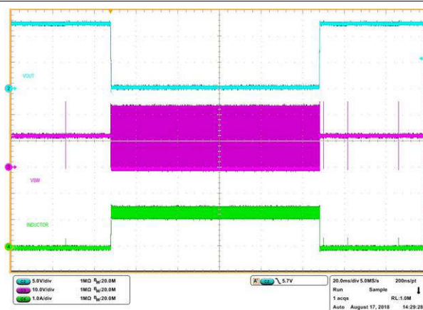
図 7-11. 短絡発生
