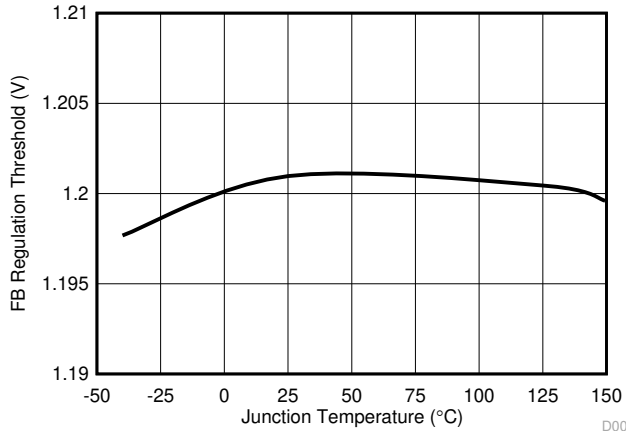
図 5-7. 帰還コンパレータ スレッシュホールドと温度との関係
