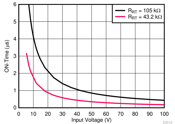
図 5-10. COT のオン時間と V_{IN} との関係
