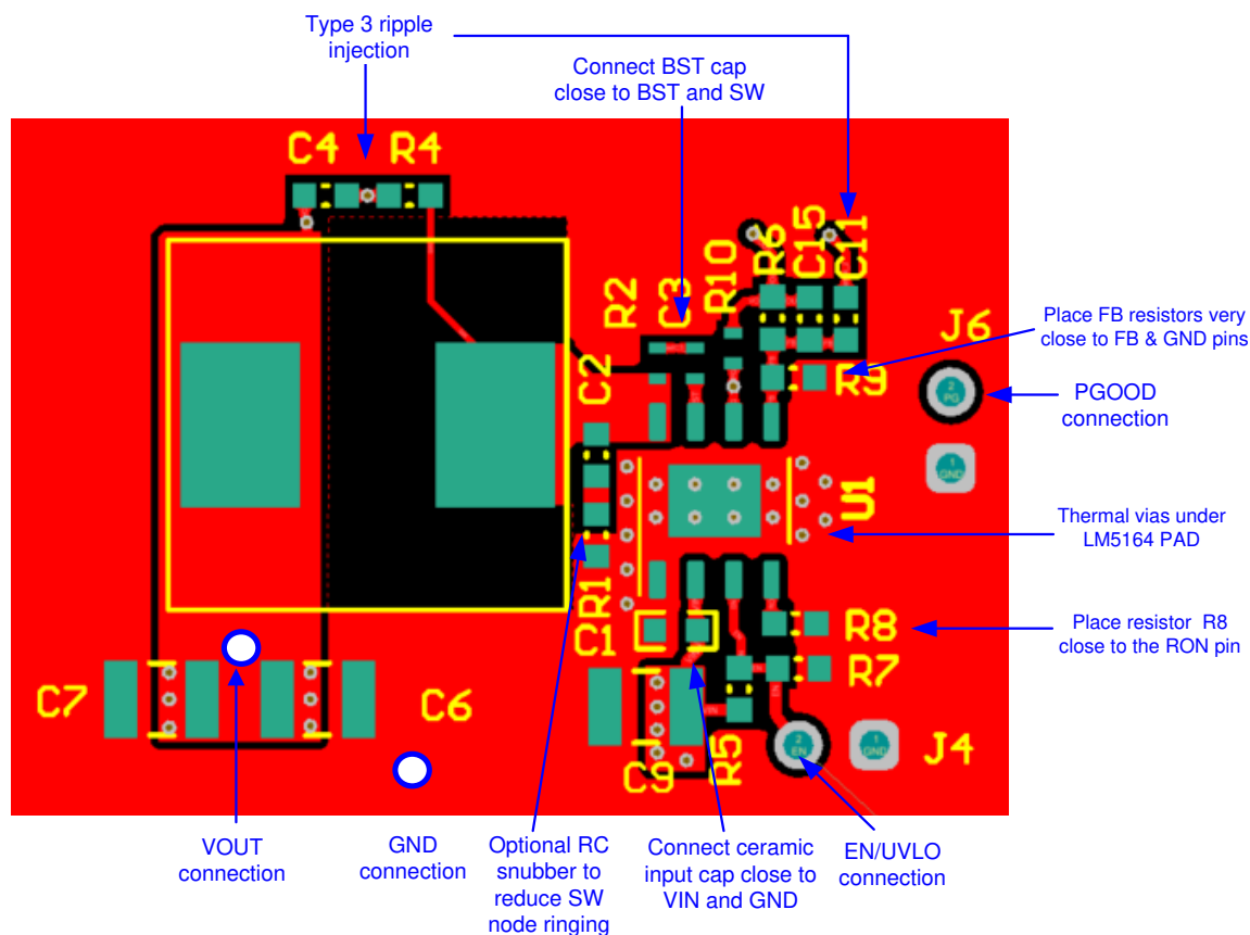
図 7-19. LM5164 片面 PCB レイアウトの例
