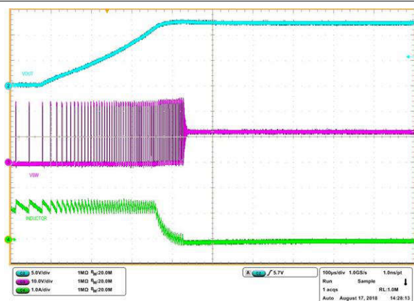
図 7-10. EN/UVLO によるプリバイアス起動
