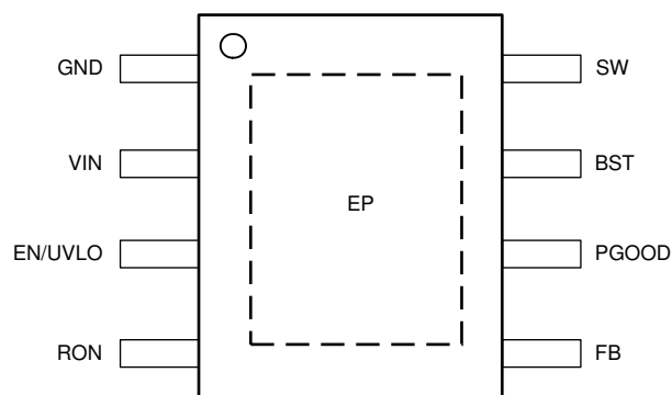
図 4-1. DDA パッケージ 8 ピン SO PowerPAD™ の IC パッケージ (上面図)
