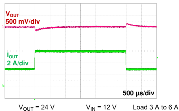
FIG 6-17. Load Step (Buck)
