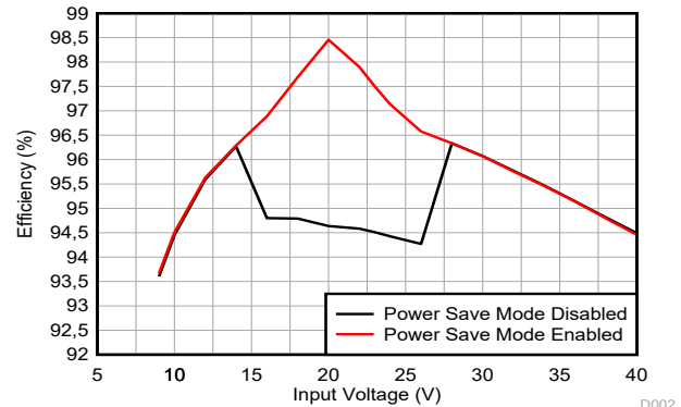
図 9-5. 効率と V_I との関係 ( V_O = 20V 、 I_O = 5A )
