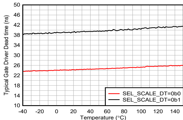
図 5-24. ゲートドライバ遷移 (デッド) 時間とスイッチング周波数との関係 f_{(sw)} = 100\text{kHz} 、SEL_MIN_DEADTIME_GDRV = 0b01、 EN_CONST_TDEAD = 0b0、ローサイド オフ、ハイサイドをオンに します
