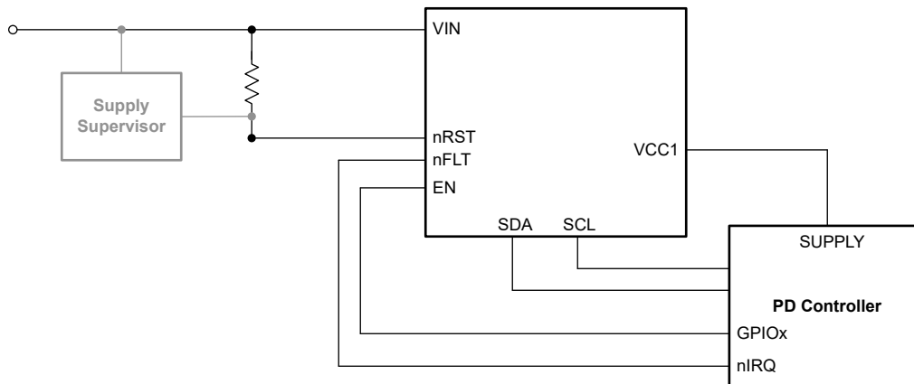
図 7-15. 概略回路図
