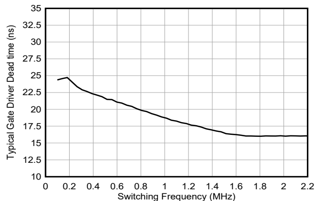
図 5-23. ゲートドライバ遷移 (デッド) 時間とスイッチング周波数との関係 SEL_MIN_DEADTIME_GDRV = 0b01、SEL_SCALE_DT = 0b0、 EN_CONST_TDEAD = 0b0
