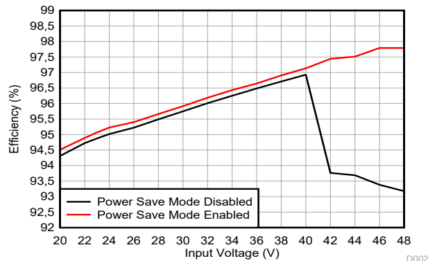
図 9-6. 効率と V_I との関係 ( V_O = 48V 、 I_O = 5A )
