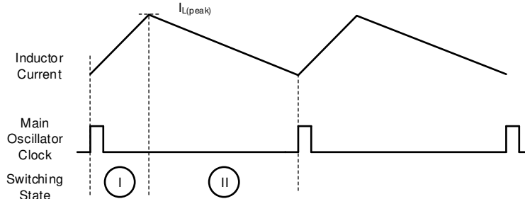
図 7-4. 連続電流昇圧動作時のインダクタ電流
