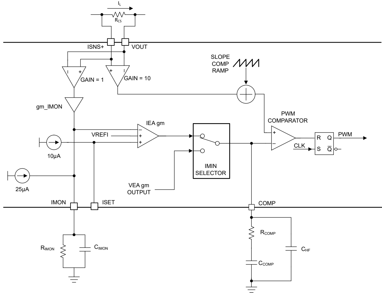
図 6-5. 電流ループの機能ブロック図
