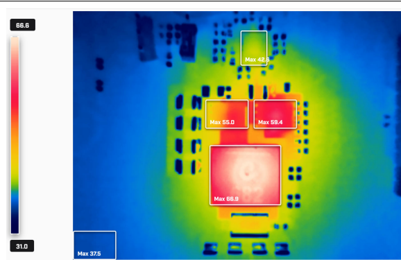
図 7-14. V_{\text{SUPPLY}} = 48\text{V} 、 I_{\text{LOAD}} = 8\text{A} 、 T_A = 25^\circ\text{C} 、エアフローなし
