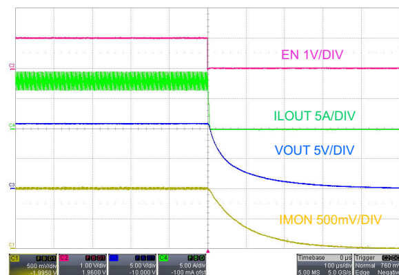
図 7-8. シャットダウン、EN オフ、V SUPPLY = 48V、 I LOAD = 8A の抵抗性負荷
