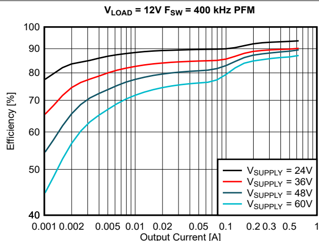
図 7-6. PFM モードの効率、対数スケール
