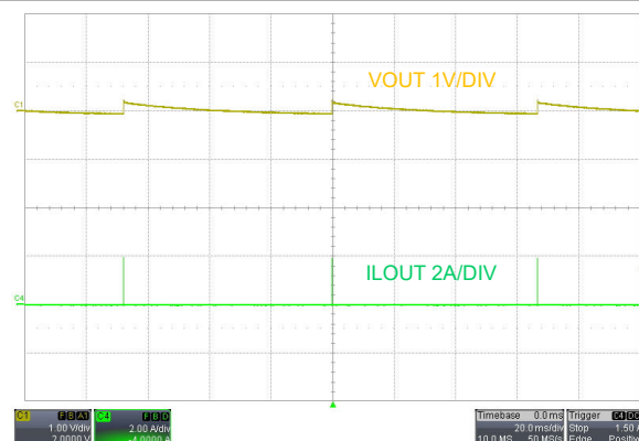
図 7-10. PFM モードでの無負荷動作、V SUPPLY = 48V、 I LOAD = 0A
