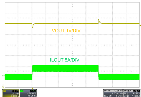
図 7-11. 負荷過渡応答、 V_{\text{SUPPLY}} = 48\text{V} 、FPWM、0A ~ 4A
