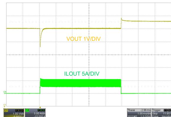
図 7-12. 負荷過渡応答、 V_{\text{SUPPLY}} = 48\text{V} 、PFM、0A ~ 4A
