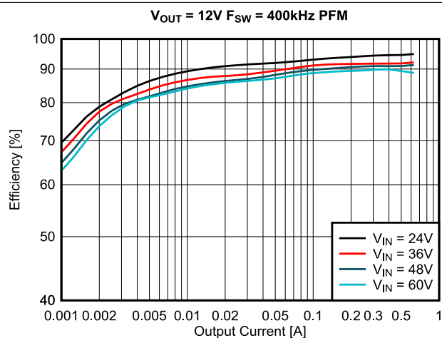
図 9-5. PFM モードの効率、対数スケール
