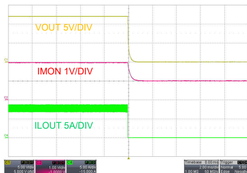
図 9-7. シャットダウン、EN オフ、 V_{SUPPLY} = 48V 、 I_{LOAD} = 8A の抵抗性負荷
