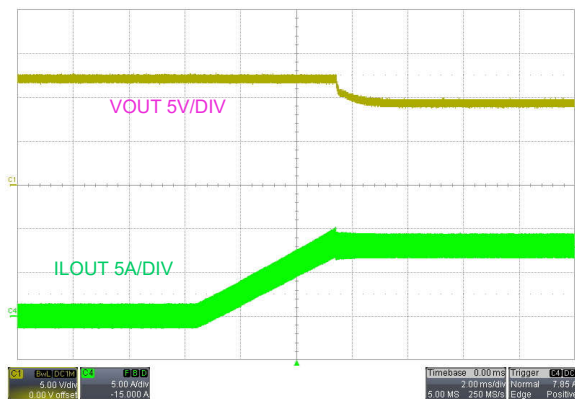
図 9-12. CV から CC モードへの遷移、 V_{\text{SUPPLY}} = 48\text{V} 、 V_{\text{LOAD}} = 12\text{V} から 9V
