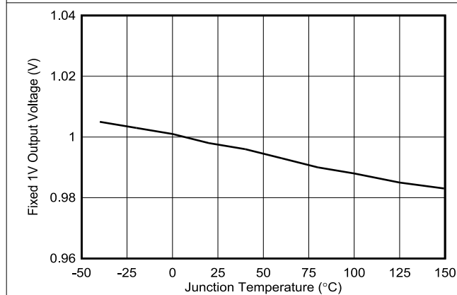
図 6-5. 固定出力電圧と温度との関係 ( V_{OUT} = 1\text{V} )
