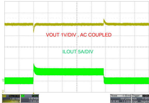
図 9-10. 負荷過渡応答、 V_{\text{SUPPLY}} = 48\text{V} 、FPWM、0A ~ 4A
