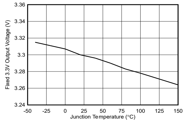
図 6-6. 固定出力電圧と温度との関係 ( V_{OUT} = 3.3\text{V} )
