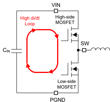
図 9-14. 入力電流ループ
