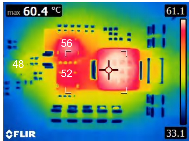
図 9-13. V_{\text{SUPPLY}} = 48\text{V} 、 I_{\text{LOAD}} = 8\text{A} 、 T_A = 25^\circ\text{C} 、エアフローなし
