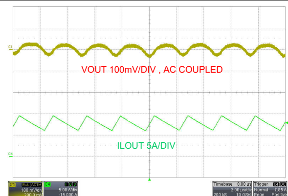
図 9-8. 出力リップル、 V_{SUPPLY} = 48V 、 I_{LOAD} = 8A
