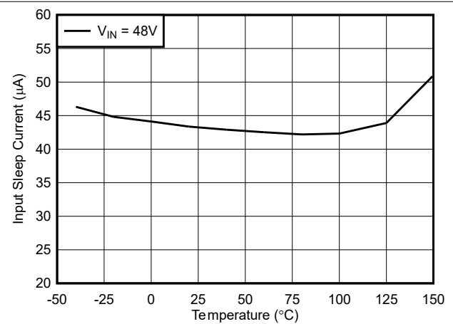
図 6-4. 入力スリープ電流と温度との関係、 V_{OUT} = 5\text{V}
