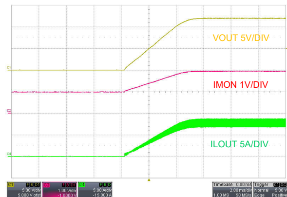
図 9-6. スタートアップ、EN オン、 V_{SUPPLY} = 48V 、 I_{LOAD} = 8A の抵抗性負荷
