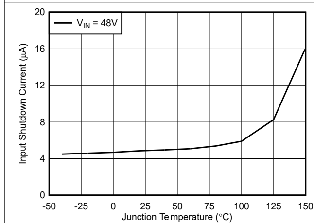
図 6-3. 入力シャットダウン電流と温度との関係
