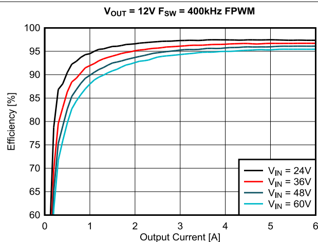
図 9-4. FPWM モードの効率、リニア スケール
