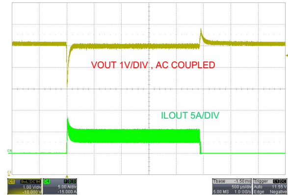
図 9-11. 負荷過渡応答、 V_{\text{SUPPLY}} = 48\text{V} 、PFM、0A ~ 4A
