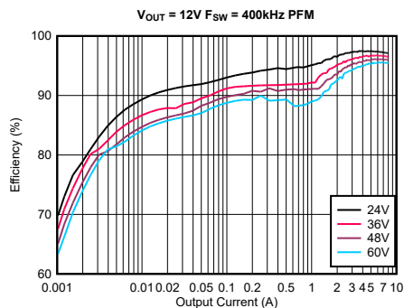
LM5192 の効率
