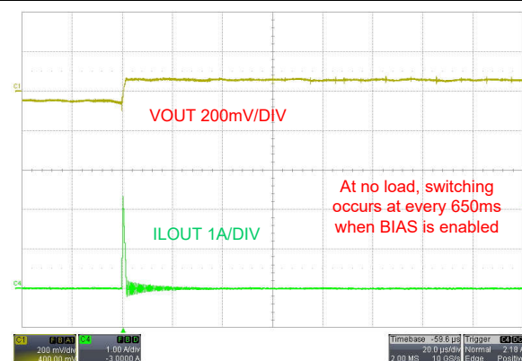
図 9-9. PFM モードでの無負荷動作、 V_{SUPPLY} = 48V 、 I_{LOAD} = 0A
