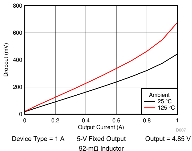
9-7. Dropout Voltage
