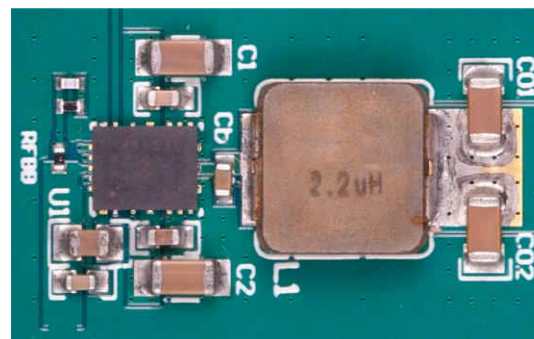
代表的な車載用のレイアウト (22mm x 12.5mm)
