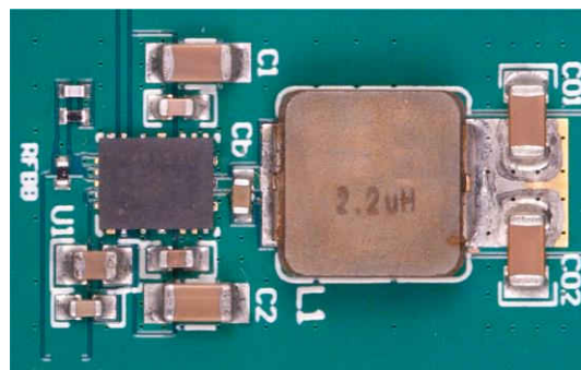
代表的な車載用のレイアウト ( 22\text{mm} \times 12.5\text{mm} )
