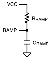
図 6-6. R RAMP to V CC for V OUT > 7.5V
