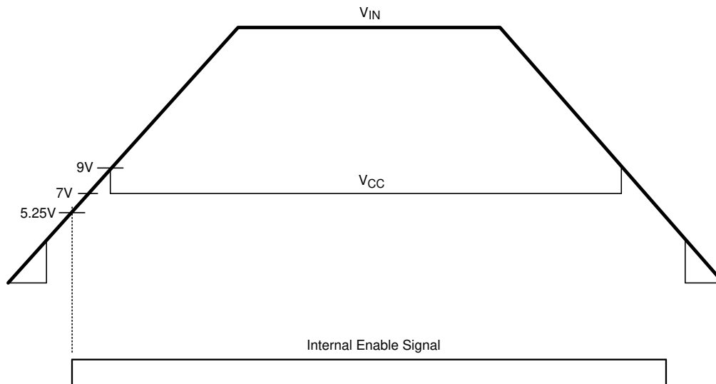
図 6-1. VIN and VCC Sequencing
