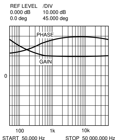
図 7-6. エラー アンプのゲインおよび位相
