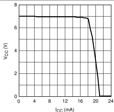
図 5-4. V_{CC} と I_{CC} V_{IN} = 12\text{V} との関係
