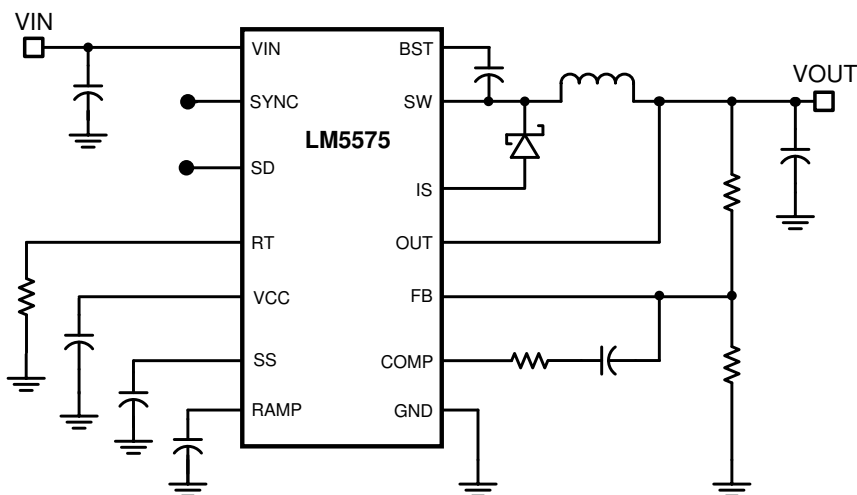
概略回路図
