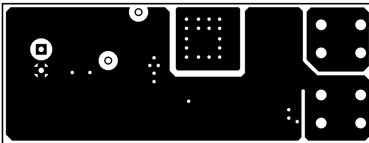
図 7-12. はんだ側
