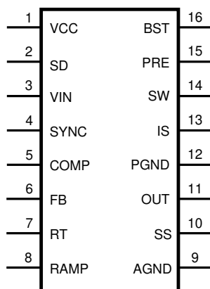
図 4-1. PWP パッケージ、16 ピン HTSSOP (露出サーマルパッド付き) (上面図)
