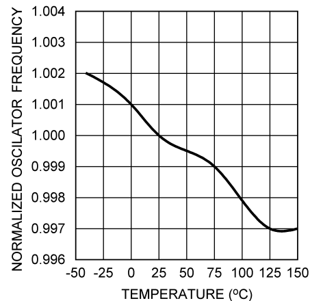
図 5-2. ( F_{OSC} = 200\text{kHz} 時)
