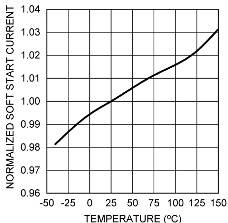
図 5-3. ソフトスタート電流と温度との関係
