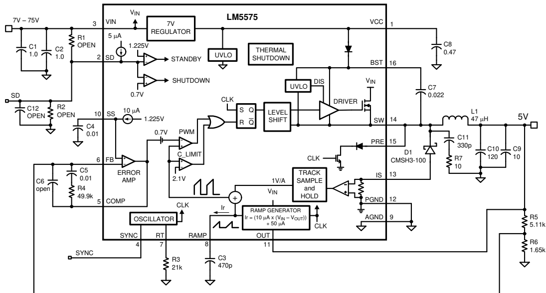
図 7-3. 代表的なアプリケーション回路
