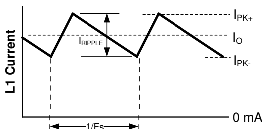
図 7-4. インダクタ電流の波形
