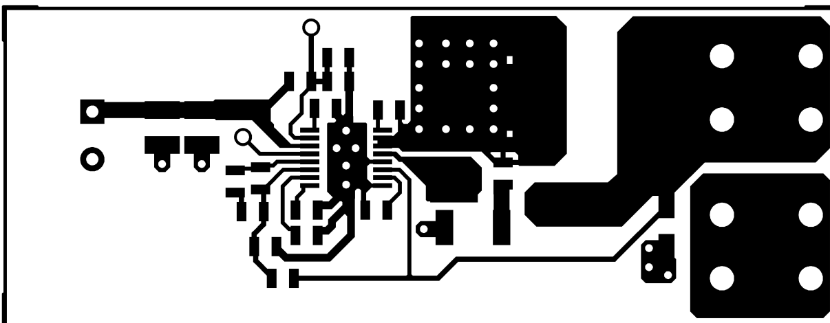
図 7-11. コンポーネント側
