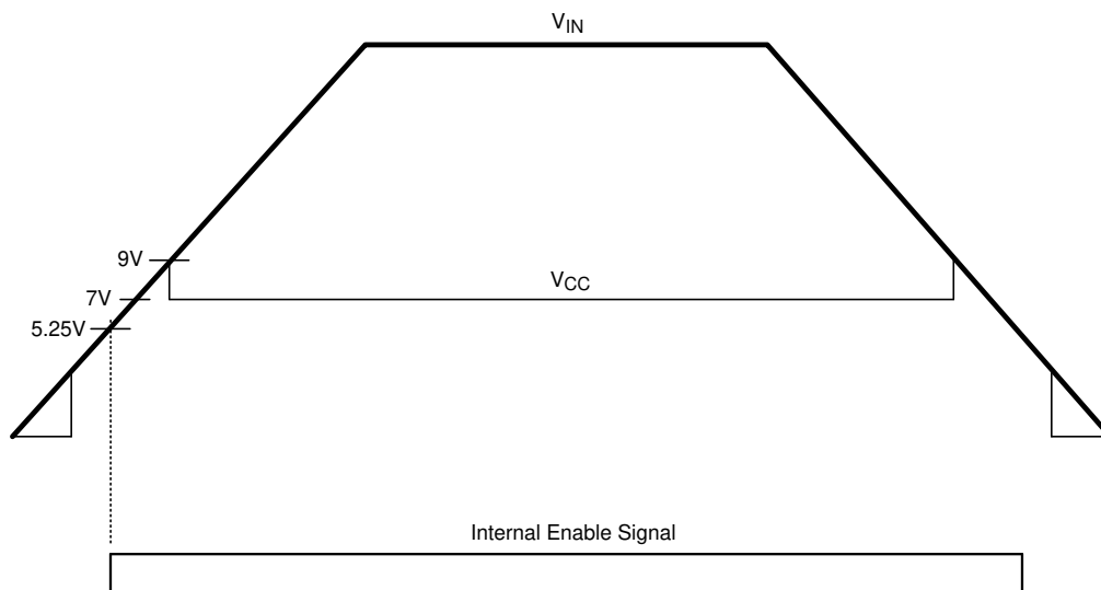
図 6-1. VIN および V CC シーケンス
