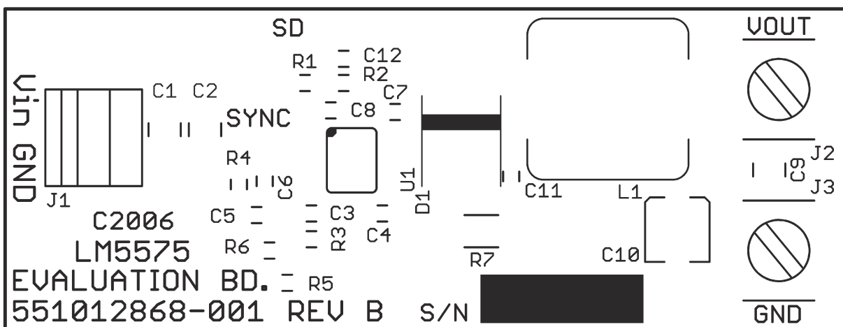
図 7-10. シルksクリーン
