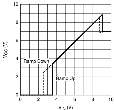
図 5-5. V_{CC} と V_{IN} R_L = 7\text{k}\Omega との関係
