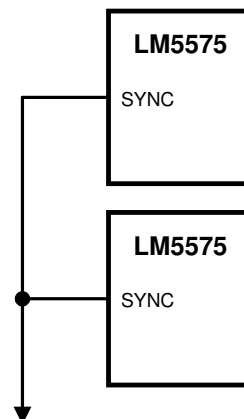
図 6-3. 複数のデバイスからの同期
