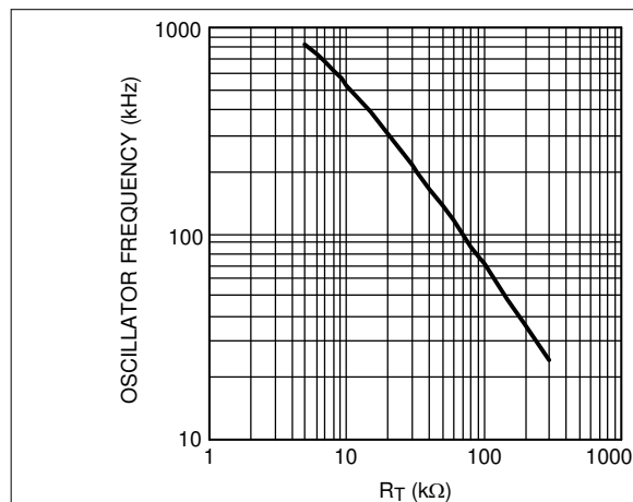
図 7-8. 発振器周波数と R_T との関係
