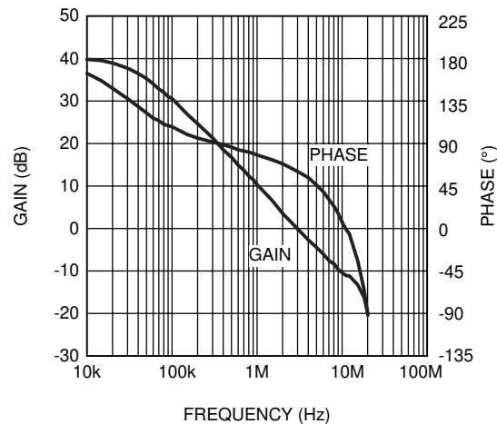
図 5-6. エラー アンプのゲイン / 位相 A_{VCL} = 101
