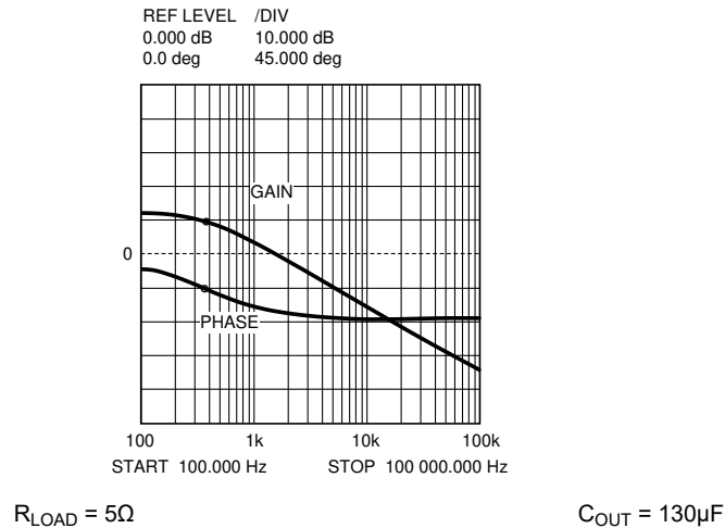
図 7-5. 変調器のゲインと位相
