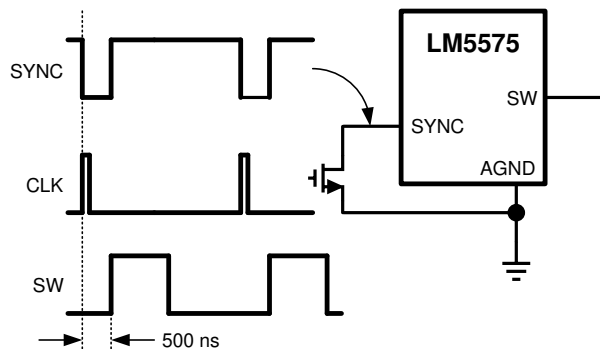
図 6-2. 外部クロックからの同期
