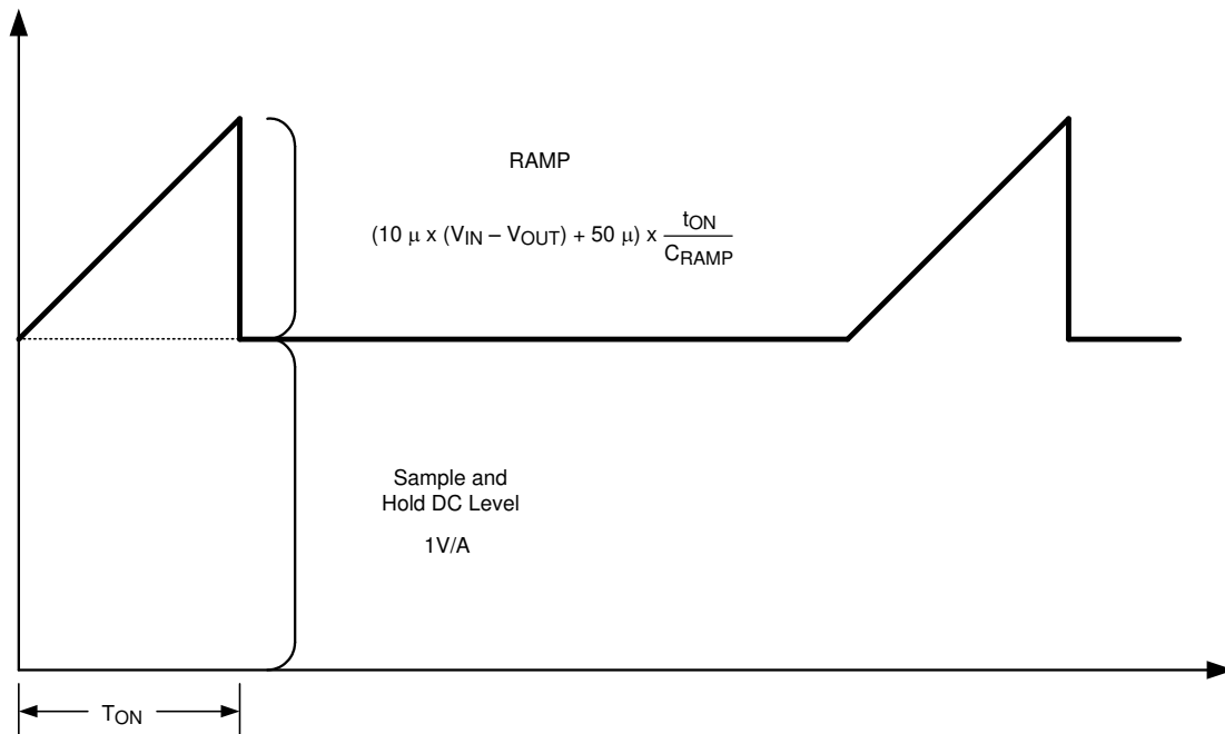
図 6-5. 電流センス信号の構成
