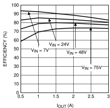
図 5-9. デモボード効率と I_{OUT} および V_{IN}
