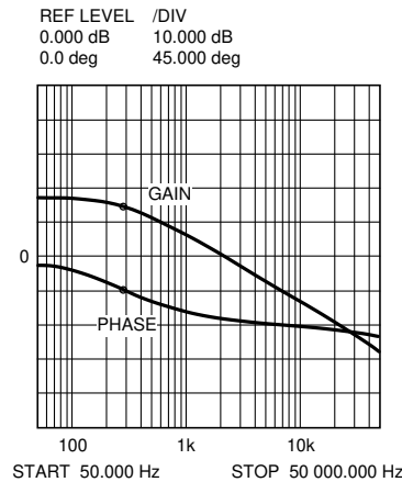
図 7-5. 変調器のゲインと位相 R = 5\Omega および C = 177\mu F 負荷アウト
