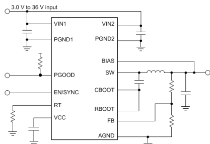
概略回路図
