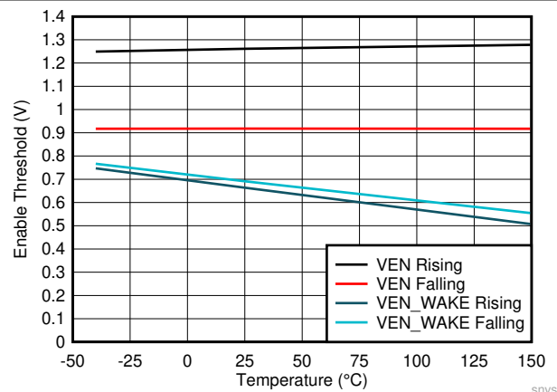
7-7. Enable Thresholds
