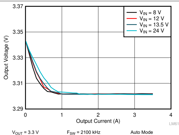
图 9-9. LM62435-Q1 Load and Line Regulation
