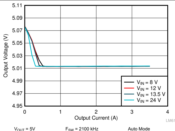
图 9-11. LM62435-Q1 Load and Line Regulation
