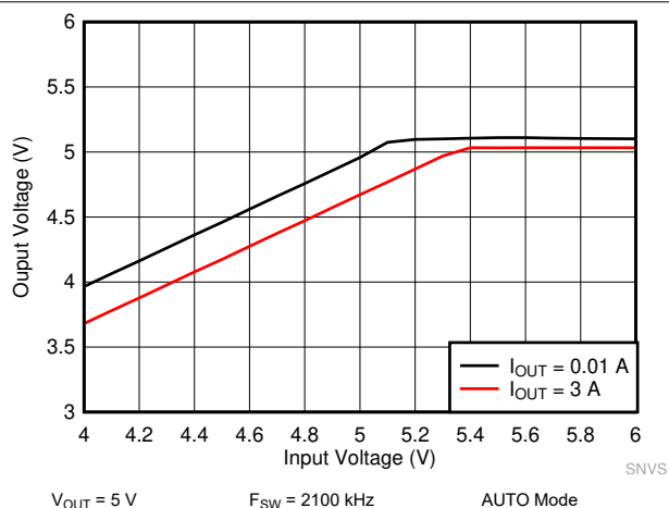
图 9-14. LM62435-Q1 Dropout Curve
