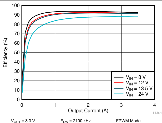
图 9-6. LM62435-Q1 Efficiency
