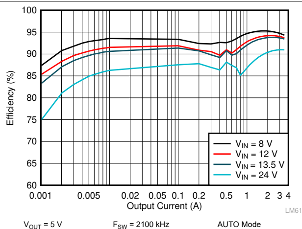
图 9-7. LM62435-Q1 Efficiency
