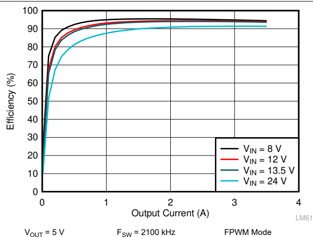
图 9-8. LM62435-Q1 Efficiency
