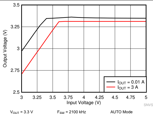
图 9-13. LM62435-Q1 Dropout Curve
