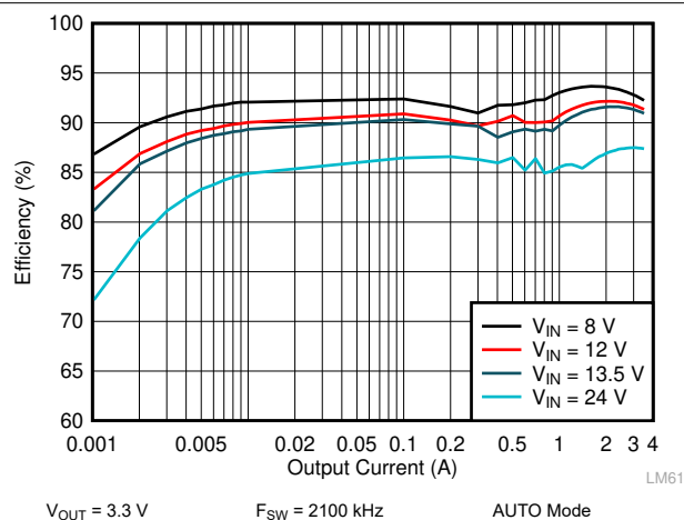
图 9-5. LM62435-Q1 Efficiency
