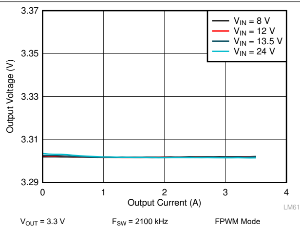
图 9-10. LM62435-Q1 Load and Line Regulation
