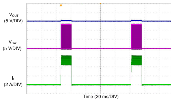
图 9-20. LM62435-Q1 Short Circuit Protection
