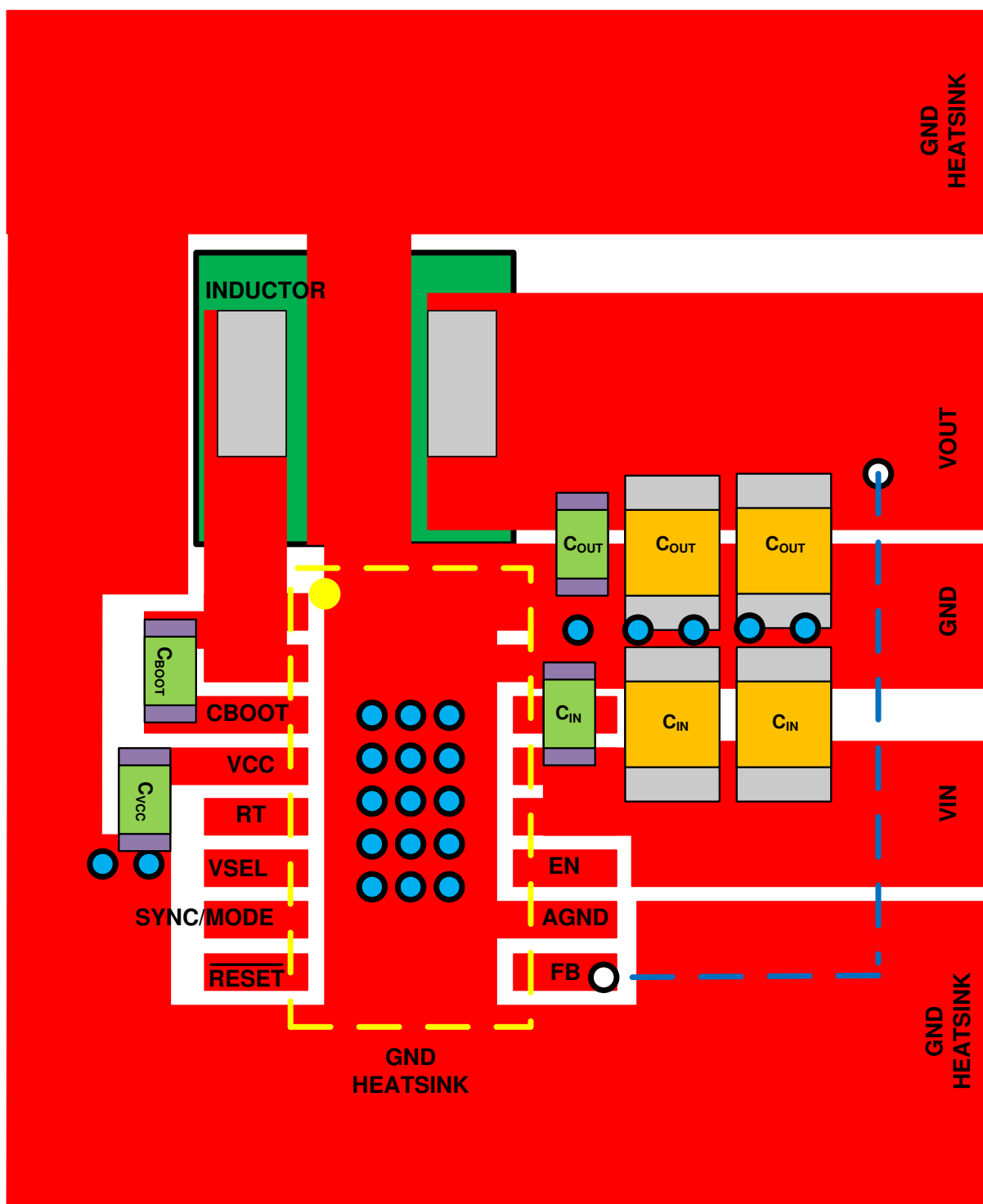
図 8-28. レイアウト例
