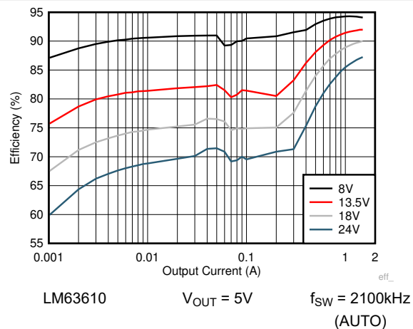
図 8-6. 効率
