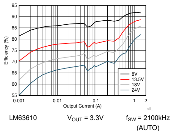
図 8-8. 効率
