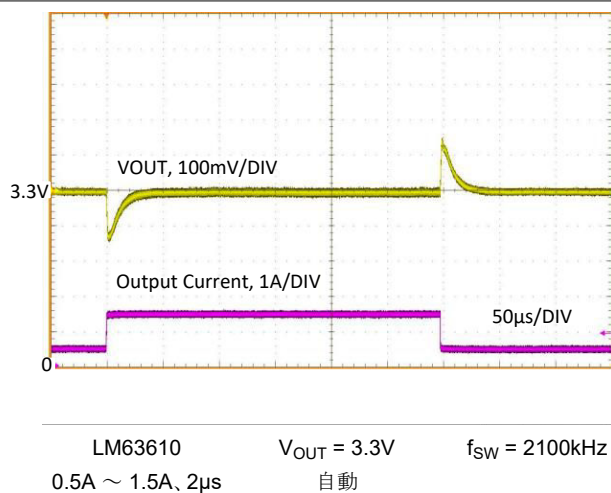
図 8-16. 負荷過渡
