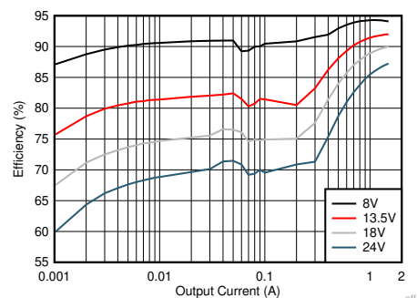
代表的な効率 ( V_{\text{out}} = 5\text{V} 、2.1MHz)
