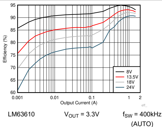
図 8-7. 効率
