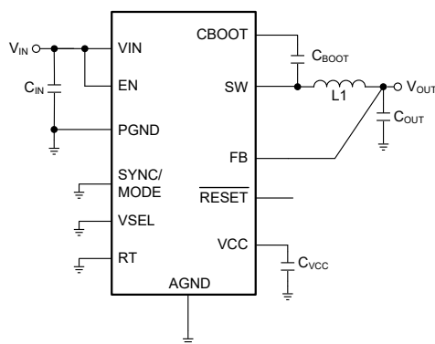
概略回路図
