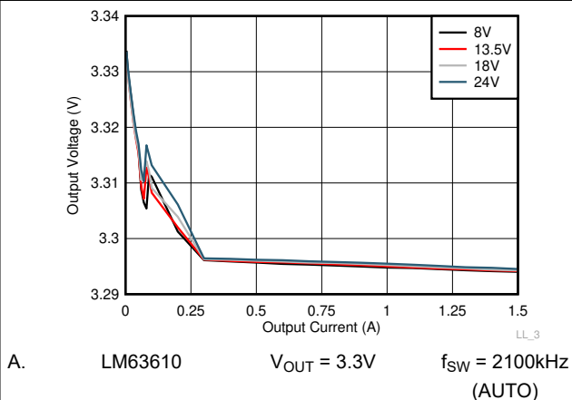
図 8-10. ライン/ロードレギュレーション
