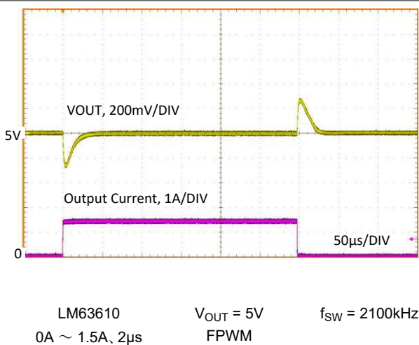
図 8-15. 負荷過渡
