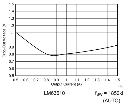
図 8-19. ドロップアウト電圧と 1.85MHz までの出力電流との関係
