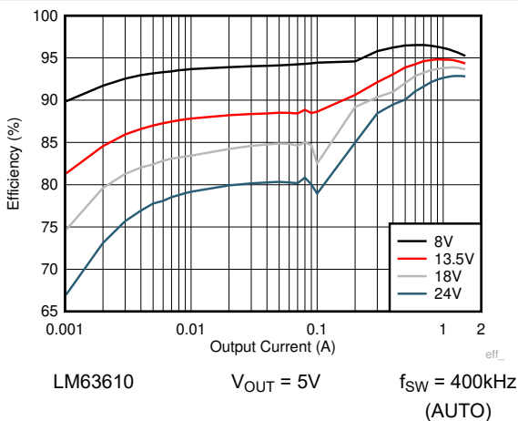
図 8-5. 効率
