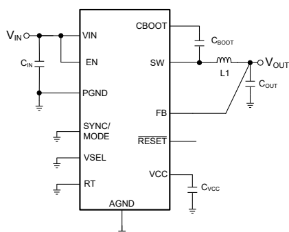
概略回路図
