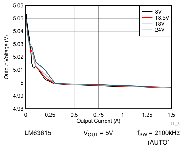
図 8-18. ラインおよびロード レギュレーション
