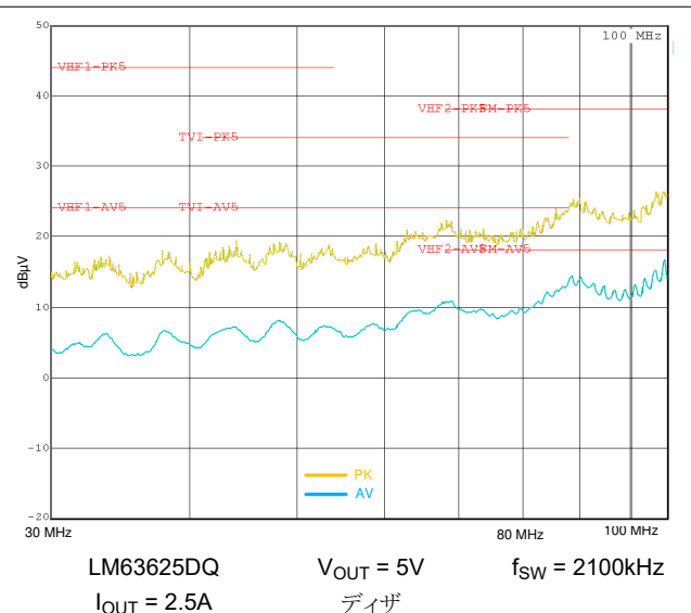
図 8-46. 30MHz ~ 108MHz の伝導型 EMI (代表値)
