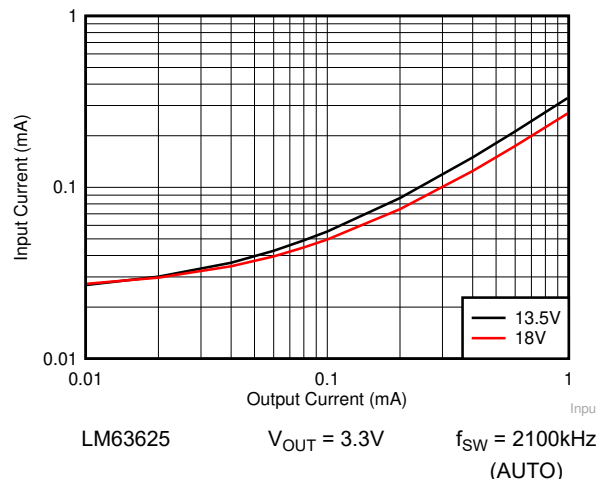
図 8-42. 入力電源電流と出力電流との関係
