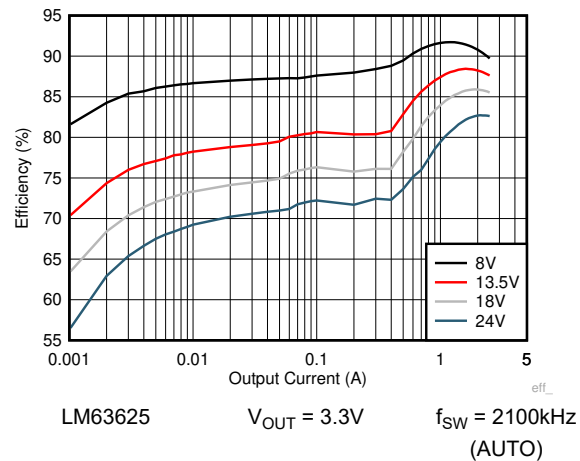
図 8-13. 効率
