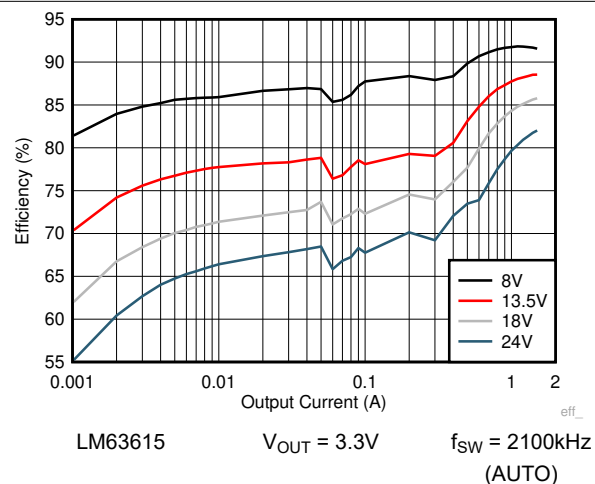
図 8-15. 効率
