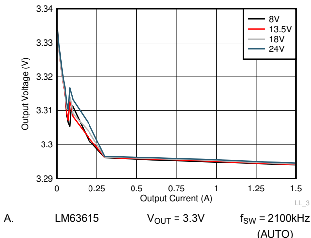
図 8-19. ラインおよびロード レギュレーション
