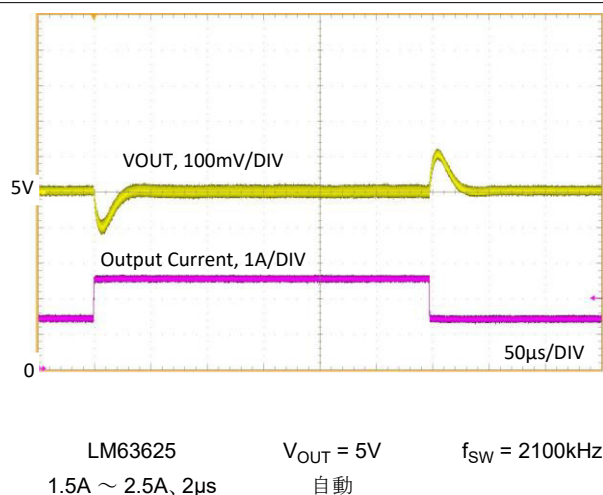
図 8-32. 負荷過渡
