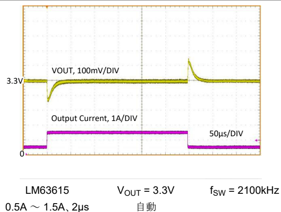
図 8-31. 負荷過渡
