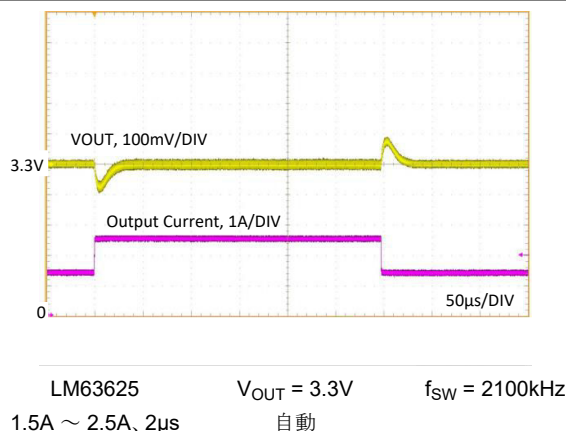
図 8-30. 負荷過渡
