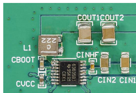
代表的な設計例、 I_{\text{OUT}} = 2.5\text{A} 、 f_{\text{SW}} = 2200\text{kHz}
