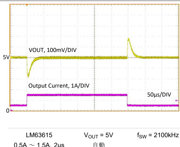
図 8-33. 負荷過渡
