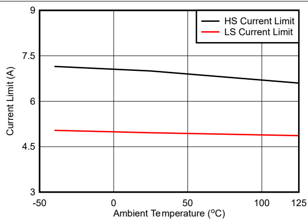
図 6-8. 4.5A 電流制限
