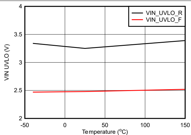
図 6-7. V_{IN} UVLO
