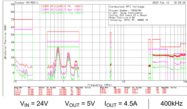
図 8-79. LM6x645 伝導 EMI - 正のライン
