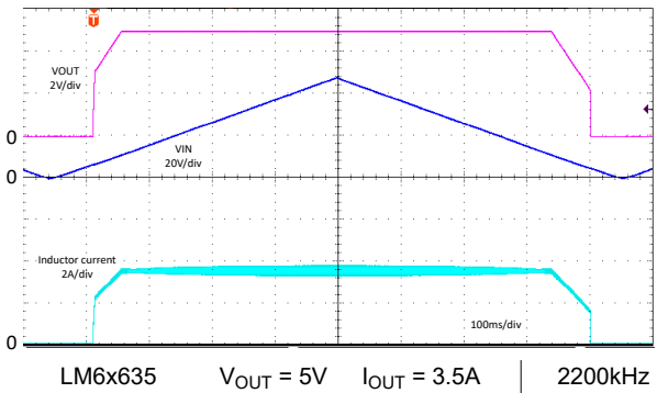
図 8-94. ライン スweep - 自動
