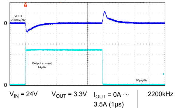
図 8-84. 負荷過渡 - LM6x635 - FPWM
