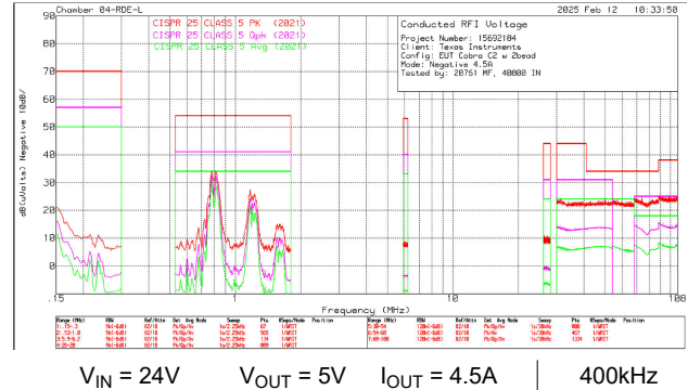
図 8-80. LM6x645 伝導 EMI - 負のライン
