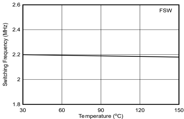
図 6-5. f_{SW} 2.2MHz
