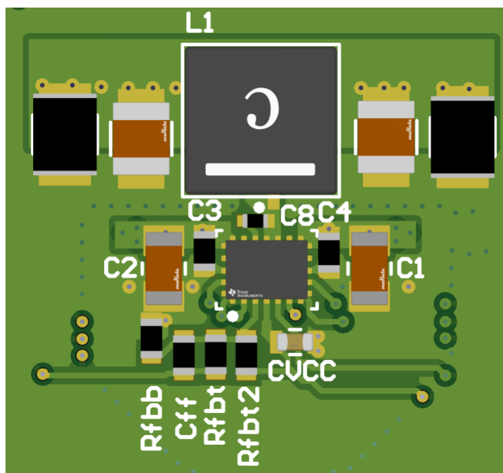
図 8-99. PCB 画像
