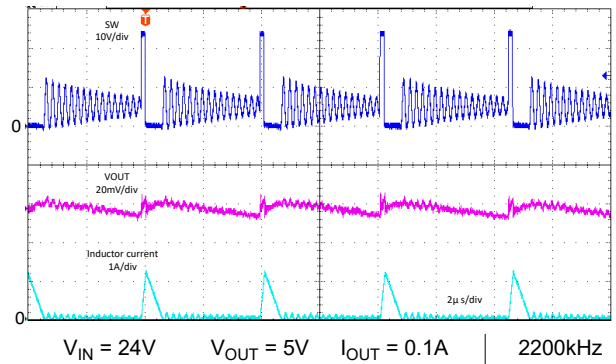
図 8-82. 代表的なスイッチング波形 - LM6x625 - 自動
