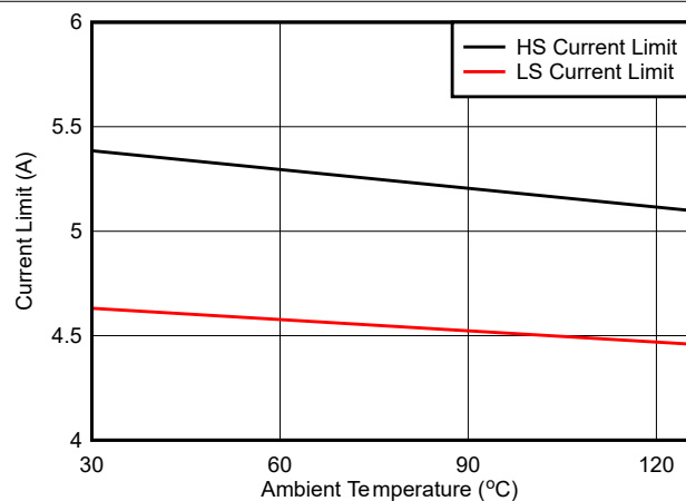
図 6-9. 3.5A 電流制限
