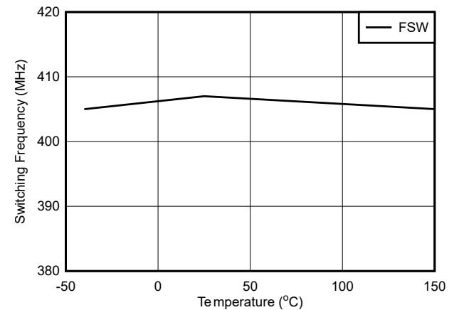
図 6-6. f_{SW} 400kHz
