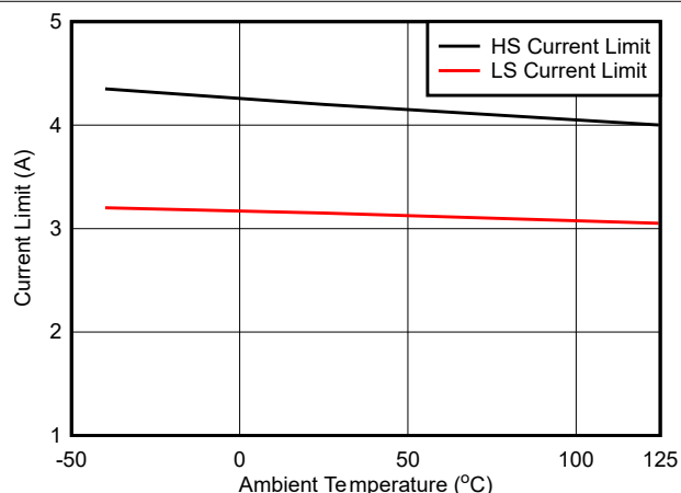
図 6-10. 2.5A 電流制限
