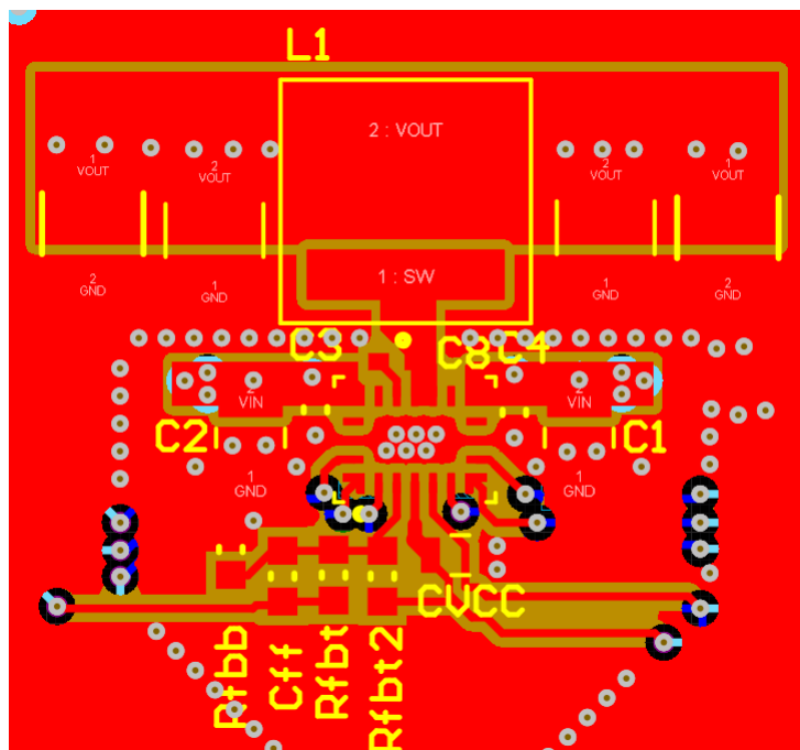
図 8-98. レイアウト例
