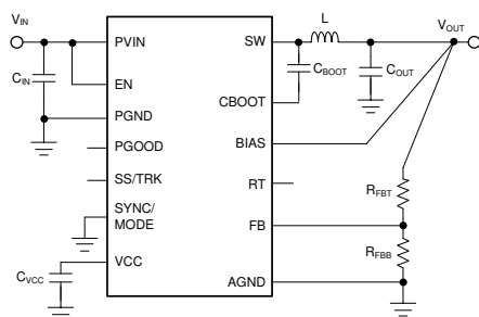
概略回路図
