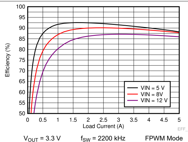
9-8. LM73605-Q1 Efficiency
