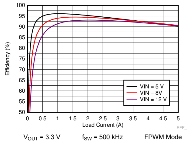
9-6. LM73605-Q1 Efficiency
