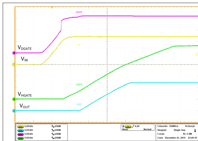
10-7. Startup 12 V with EN Pulled to VIN
