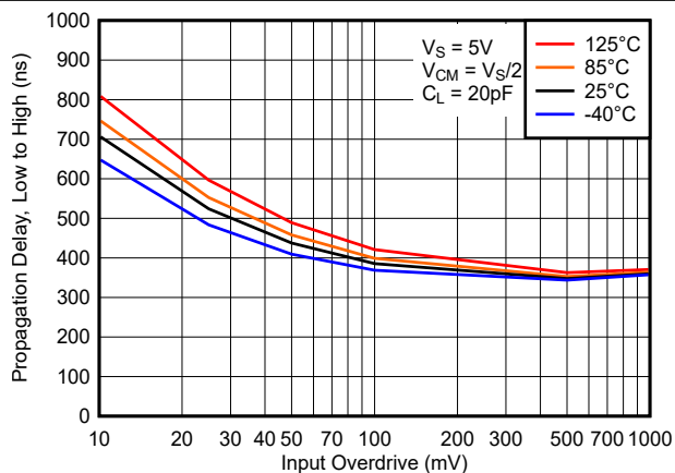
図 4-8. 伝搬遅延、"Low" から "High", 5V
