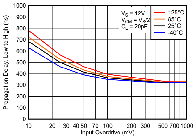
図 4-10. 伝搬遅延、"Low" から "High", 12V
