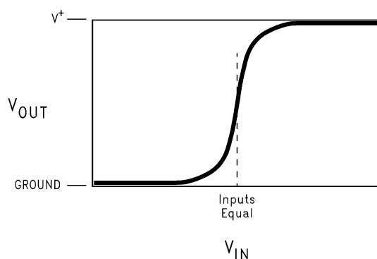
図 5-3. 正の帰還なし (ヒステリシスなし)
