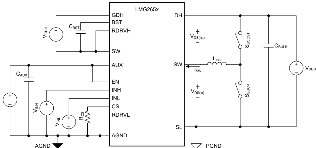
6-1. GaN Power FET Switching Parameters Test Circuit
