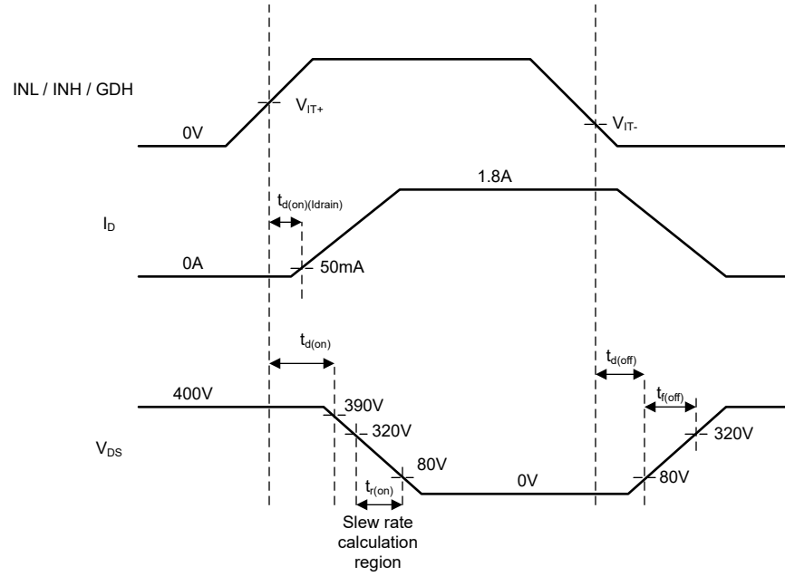
図 6-2. GaN Power FET Switching Parameters
