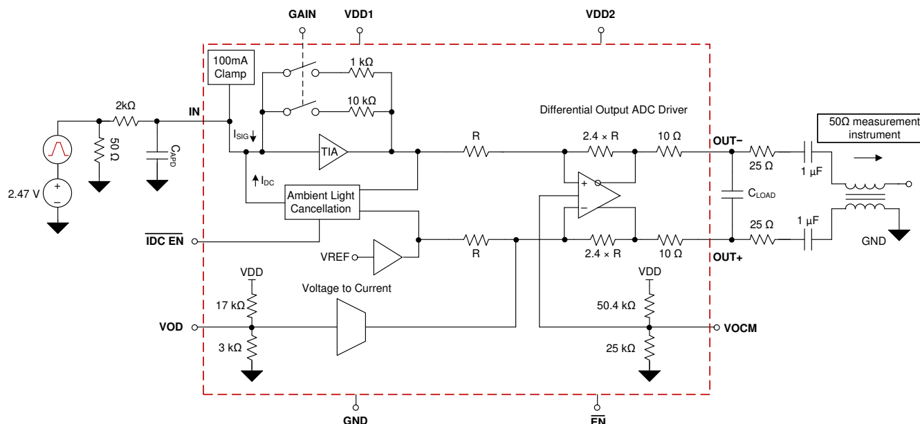
图 8-3. LMH32401 测试电路
