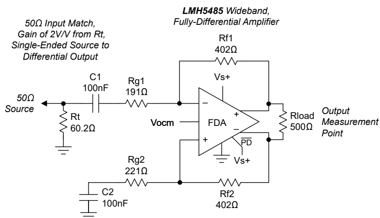
概略回路図
