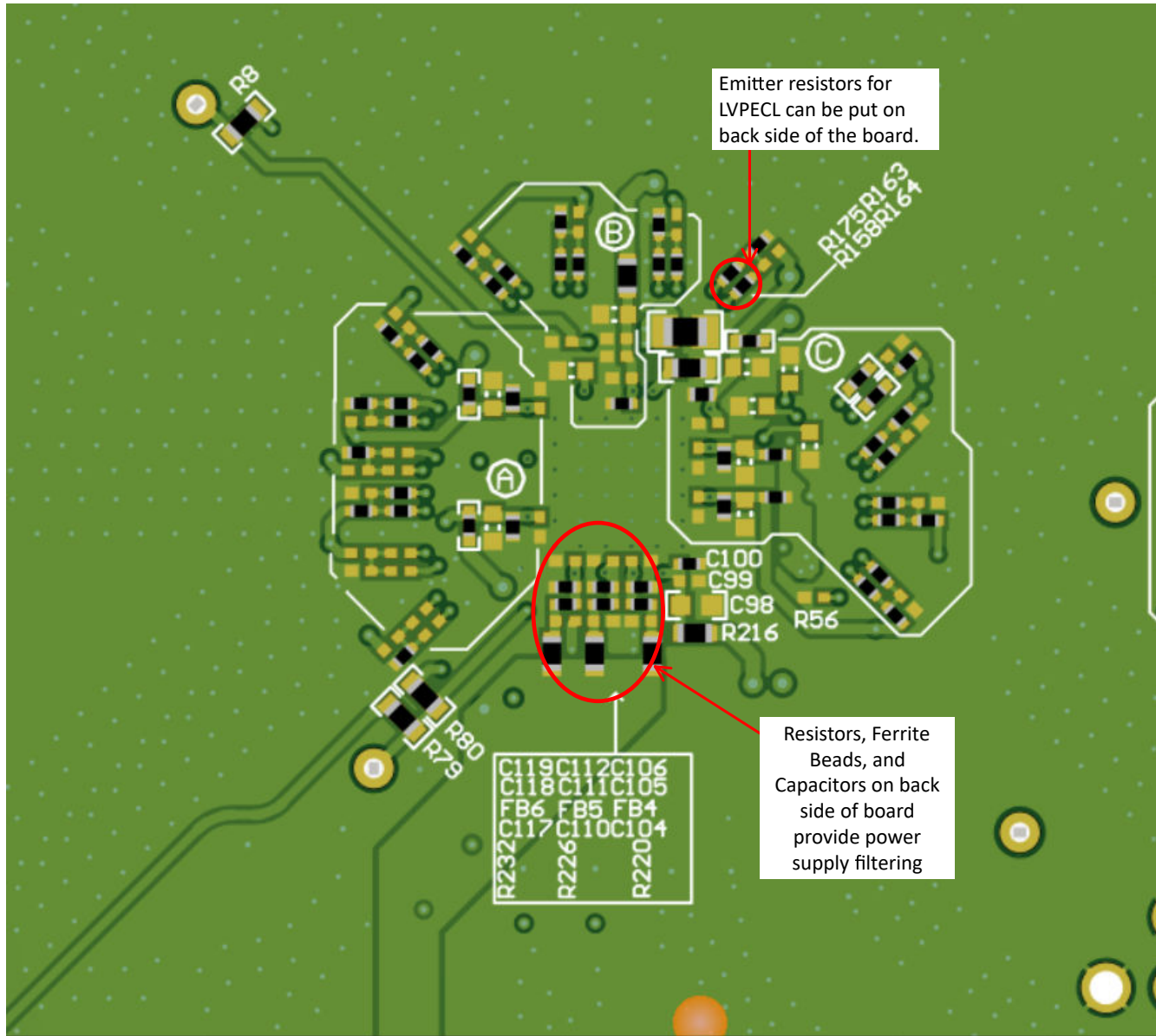
图 9-11. Bottom Layer
