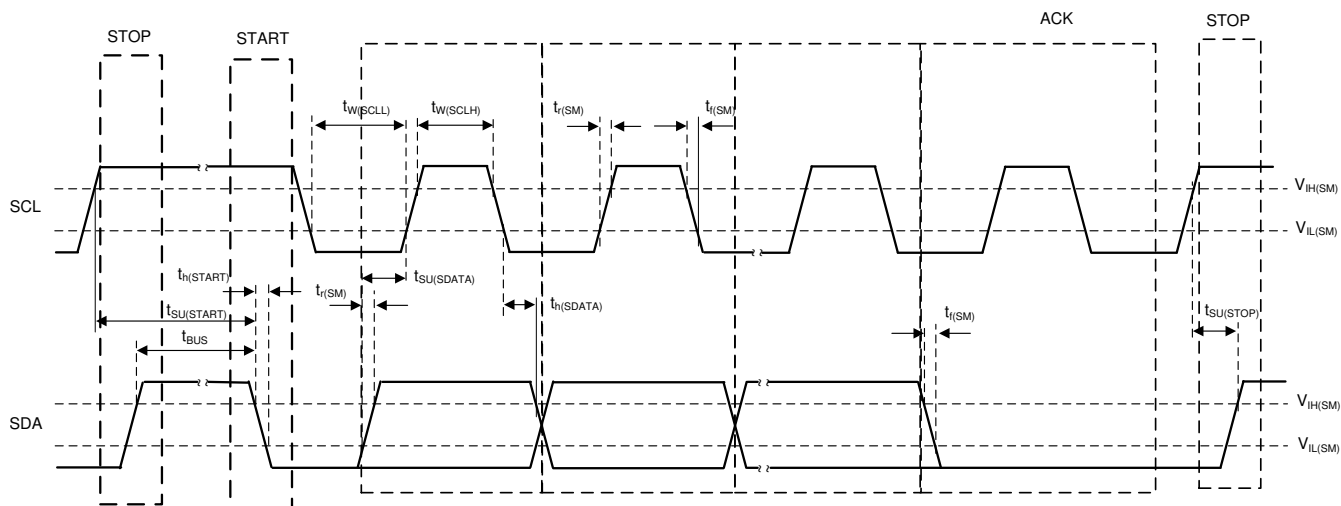
图 5-2. I²C Timing Diagram
