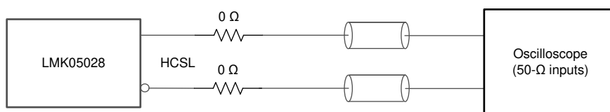
図 6-5. HCSL Output Test Configuration
