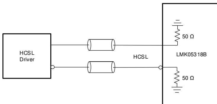
図 8-12. リファレンス (PRIREF/ SECREF) または XO 入力への DC 結合 CML (ソース終端)
