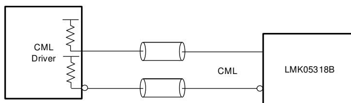
図 8-11. リファレンス (PRIREF/SECREF) または XO 入力への DC 結合 LVDS
