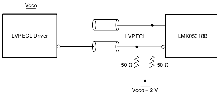
図 8-10. リファレンス (PRIREF_P/ SECREF_P) または XO 入力への DC 結合 LVPECL
