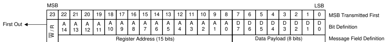
図 8-39. SPI メッセージ形式
