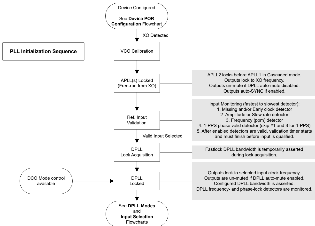
図 8-33. PLL の起動シーケンス
