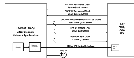
代表的なシステム ブロック図
