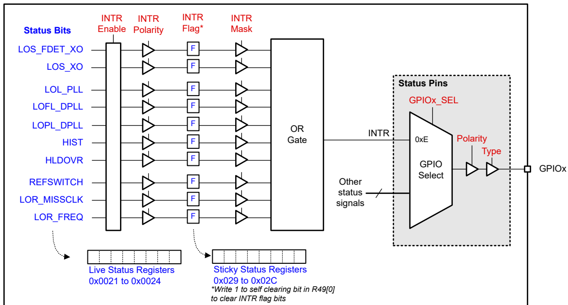
図 7-22. ステータスと割り込み
