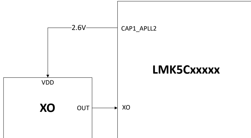
図 8-3. CAP1_APLL2 による XO 入力の供給
