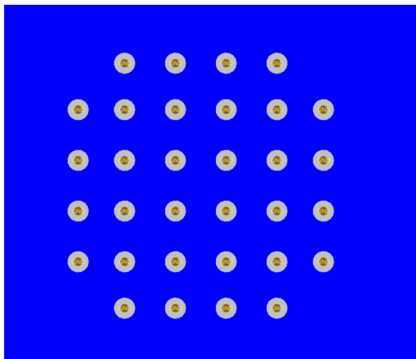
図 8-7. LMK5C22212A の PCB レイアウト例、最下層
