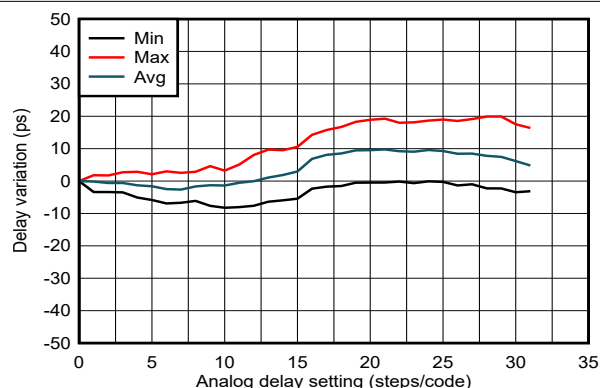
図 5-18. SYSREF/1PPS 遅延の直線性とアナログ遅延コード 3 の関係
