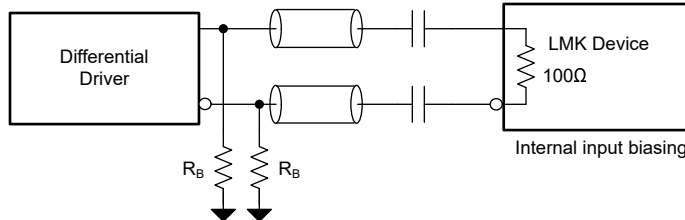
図 7-15. AC 結合差動リファレンス (INx)
