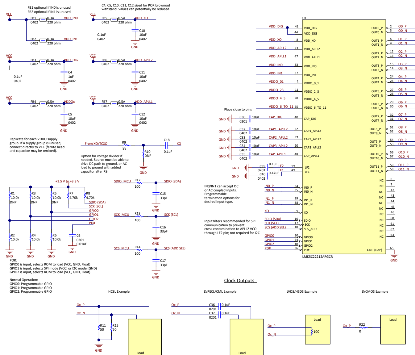
図 8-4. リファレンス回路図の例
