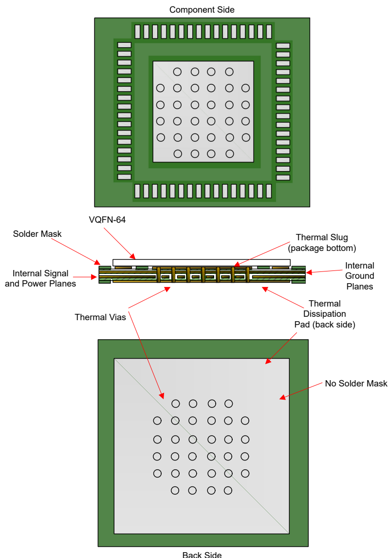
図 8-8. 熱信頼性のための一般的な PCB グランドレイアウト (8 層以上を推奨)
