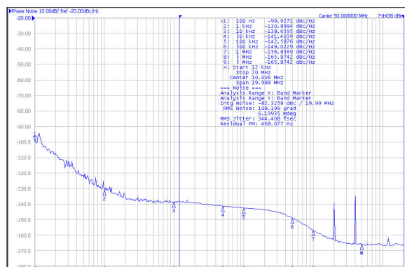
図 6-19. 50MHz HSDS Output From APLL1
