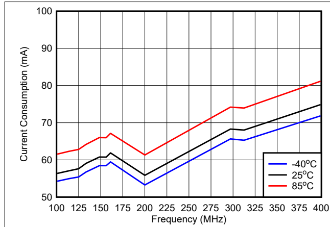
図 6-13. 消費電流と周波数との関係 (LVDS、2.5V)
