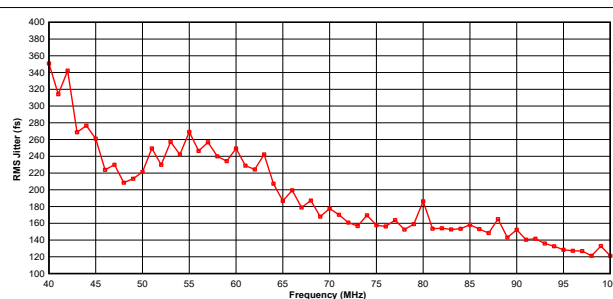
図 6-22. LVDS の RMS ジッタと周波数との関係 (100MHz 未満)、標準 3.3V、25°C
