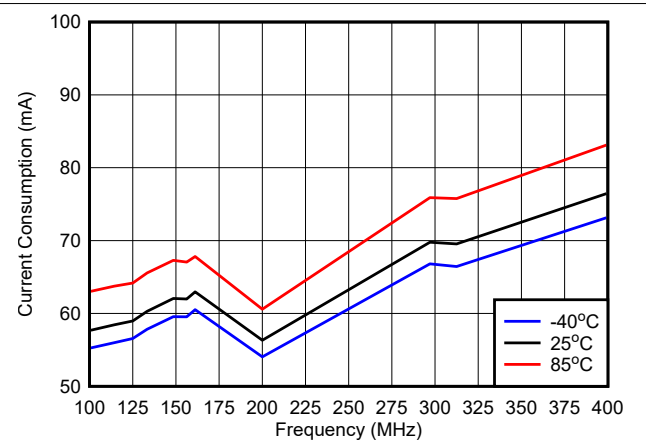
図 6-14. 消費電流と周波数との関係 (LVDS、3.3V)
