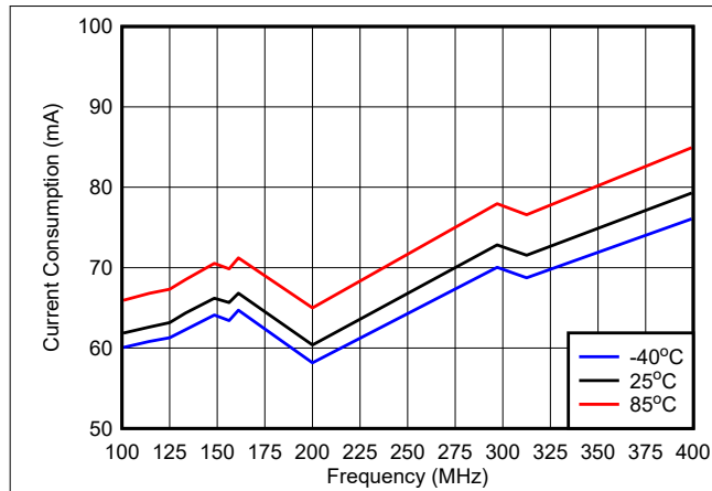
図 6-7. 消費電流と周波数との関係 (HCSL、2.5V)
