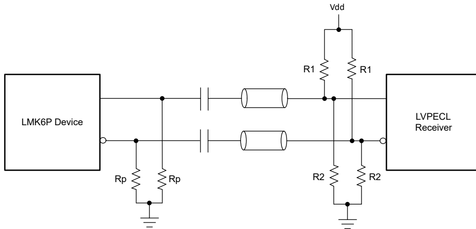
図 8-6. LVPECL レシーバに AC 結合する LMK6P 出力、外部終端 / バイアス付き (T ネットワーク)
