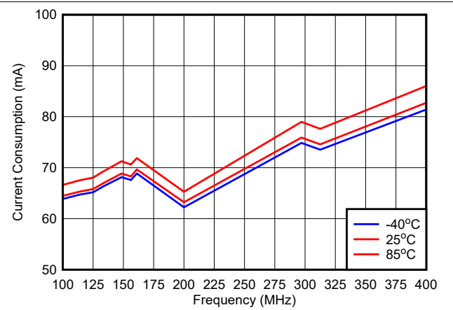
図 6-10. 消費電流と周波数との関係 (LVPECL、2.5V)
