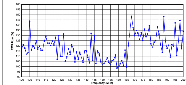
図 6-15. LVPECL、HCSSL の RMS ジッタと周波数との関係 (100MHz ~200MHz)、標準 3.3V、25°C
