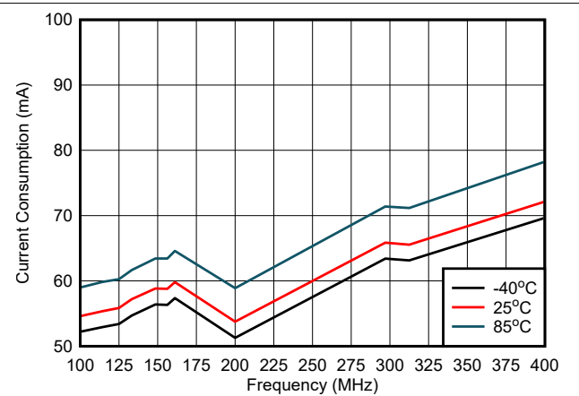
図 6-12. 消費電流と周波数との関係 (LVDS、1.8V)
