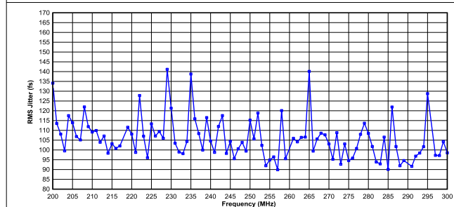
図 6-17. LVPECL、HCSSL の RMS ジッタと周波数との関係 (200MHz ~300MHz)、標準 3.3V、25°C
