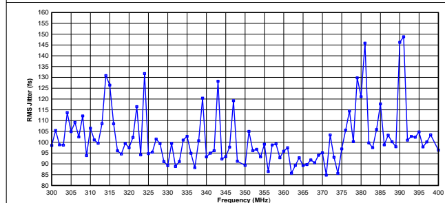
図 6-19. LVPECL、HCSSL の RMS ジッタと周波数との関係 (300MHz ~400MHz)、標準 3.3V、25°C
