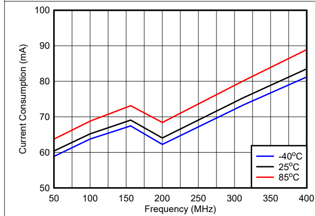
図 6-9. 消費電流と周波数との関係 (LVPECL、1.8V)
