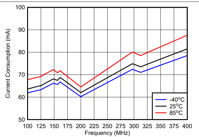
図 6-8. 消費電流と周波数との関係 (HCSL、3.3V)
