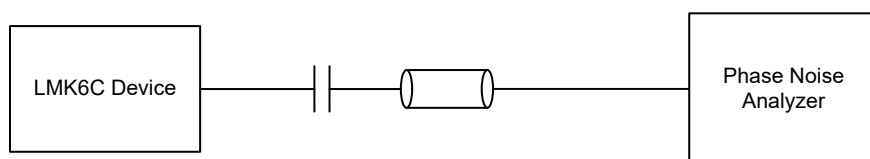
図 7-2. LMK6C の出力位相ノイズテスト構成
