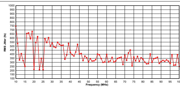
図 6-24. LVC MOS の RMS ジッタと周波数との関係 (10MHz~100MHz)、標準 3.3V、25°C
