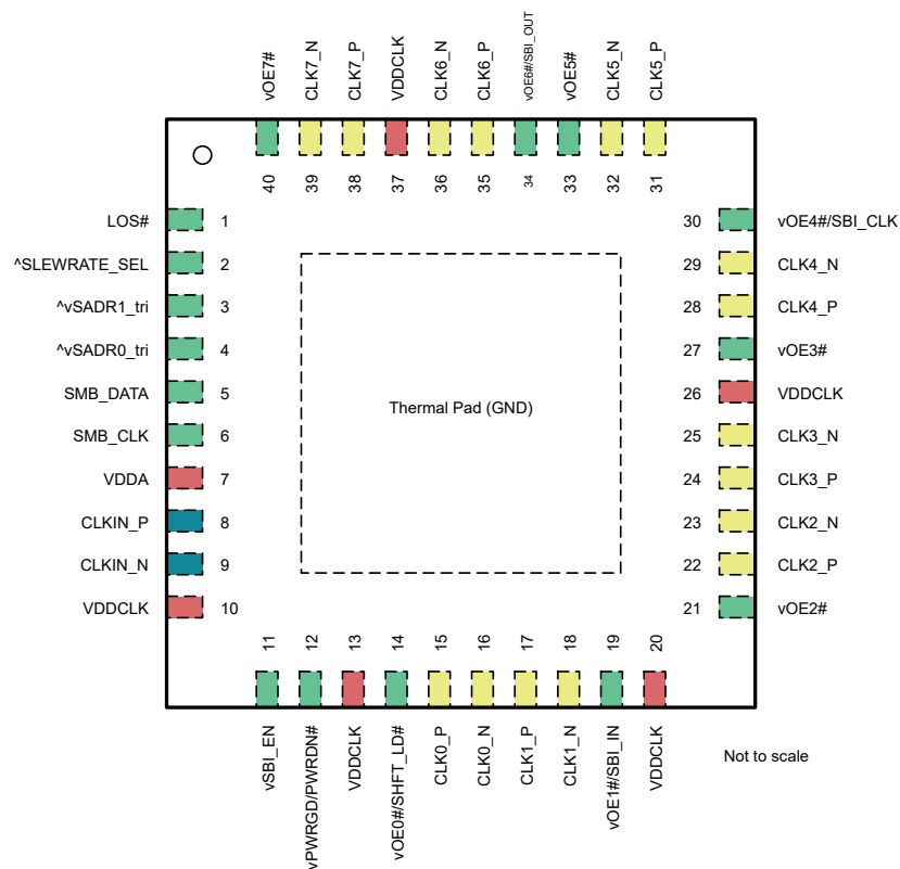
図 5-4. LMKDB1108 および LMKDB1108FS 5mm x 5mm VQFN パッケージ 40 ピン 上面図
