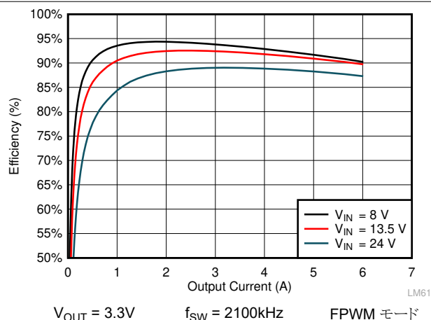
図 8-8. LMQ61460 の効率
