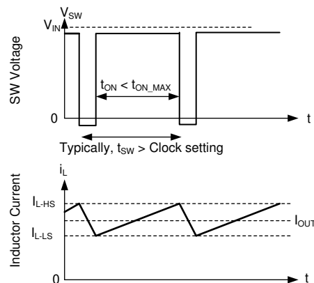
図 7-12. 電流制限波形
