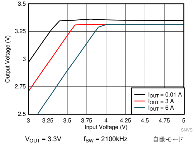
図 8-22. LMQ61460 のドロップアウト曲線
