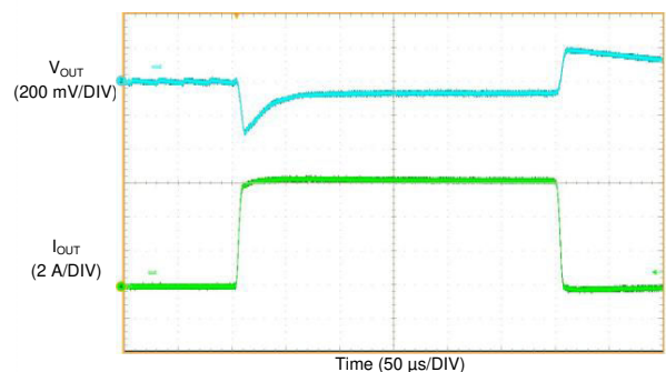
図 8-39. LMQ61460 の負荷過渡応答
