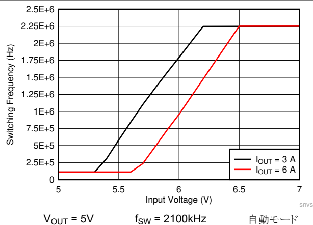
図 8-28. LMQ61460 の周波数ドロップアウト曲線
