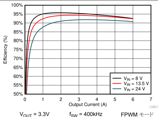
図 8-6. LMQ61460 の効率
