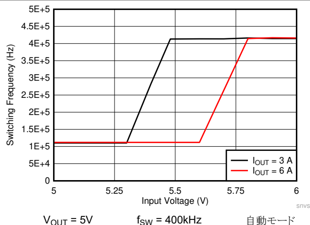
図 8-27. LMQ61460 の周波数ドロップアウト曲線
