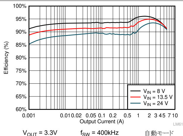
図 8-5. LMQ61460 の効率
