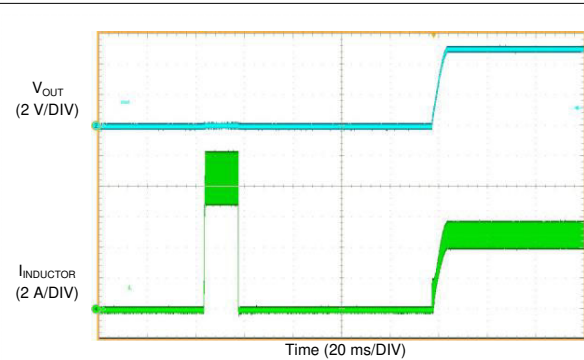
図 7-14. 短絡からの回復
