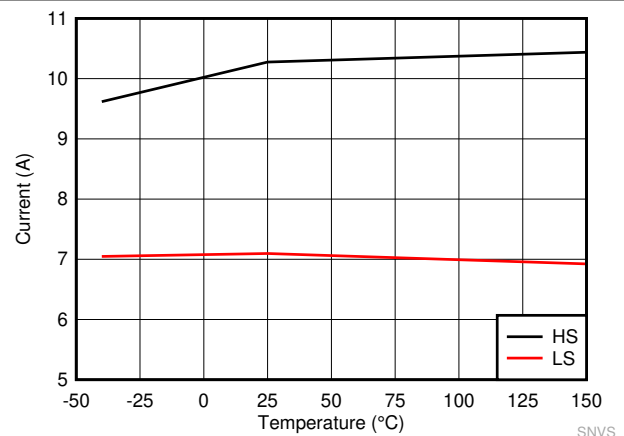
図 6-4. LMQ61460 のハイサイドおよびローサイド電流制限
