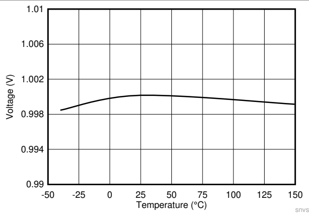
図 6-3. 帰還電圧
