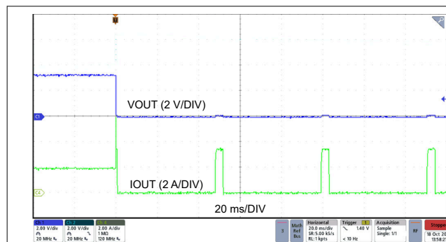
図 7-11. ヒカップの入口
