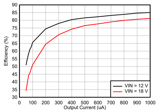
LMQ66430R5R V_{OUT} = 5V 400kHz (自動) 固定
