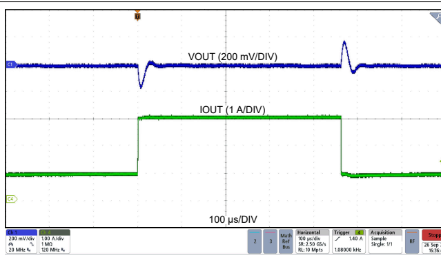
LMQ66430R5R V_{OUT} = 5V 400kHz (自動) 1A ~ 3A, 1A/ \mu s 固定
