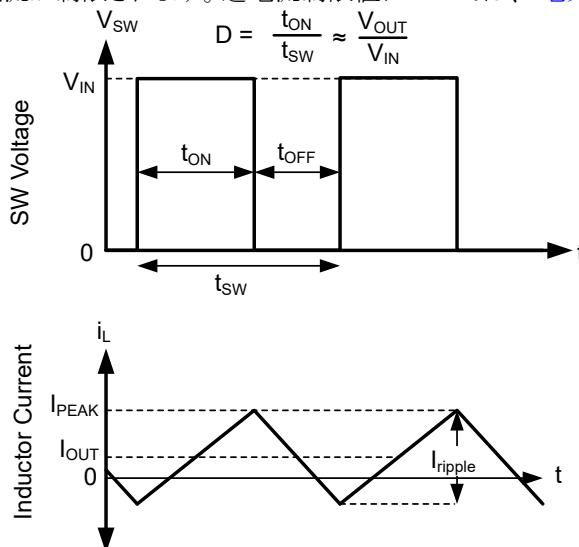
図 7-16. FPWM モード動作
