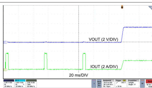
図 7-12. ヒカップの出口
