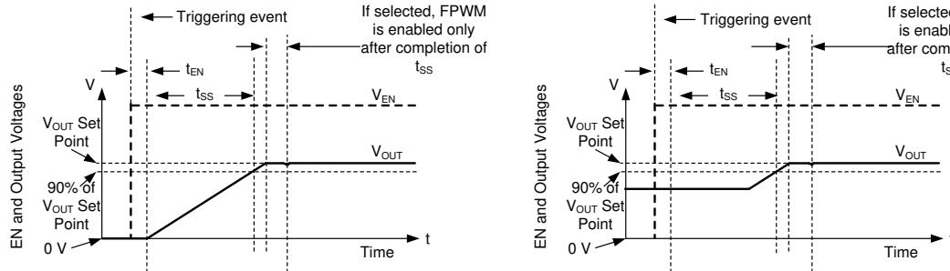
図 7-7. プリバイアス電圧の有無によるソフトスタート
