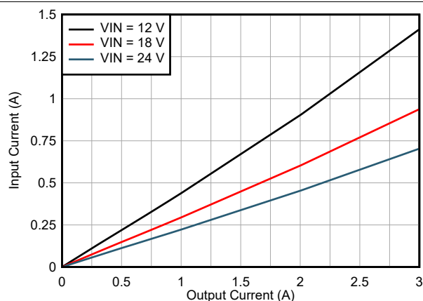
LMQ66430R5R V_{OUT} = 5V 400kHz (自動) 固定
