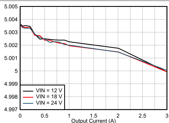
LMQ66430R5R V_{OUT} = 5V 400kHz (自動) 固定
