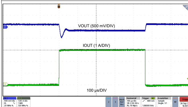
LMQ66430R5R V_{OUT} = 5V 400kHz (自動) 0A ~ 3A, 1A/ \mu s 固定
