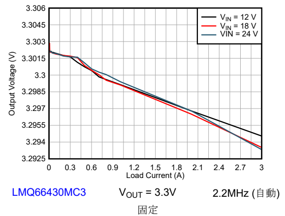
図 8-7. ラインレギュレーションおよびロードレギュレーション
