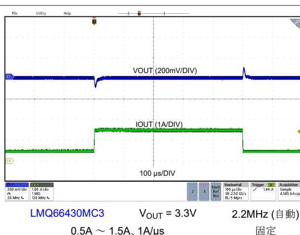
図 8-11. 負荷過渡
