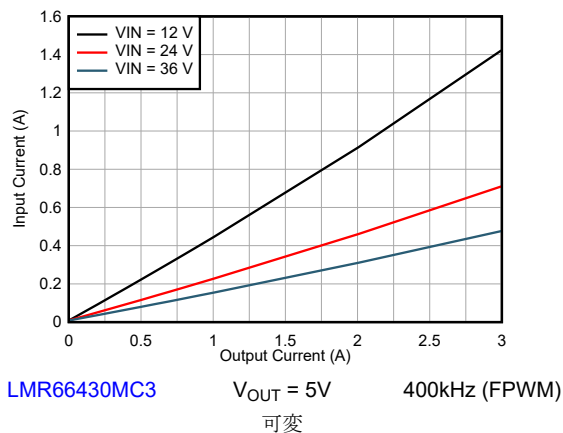
図 8-29. 入力電流と負荷電流との関係
