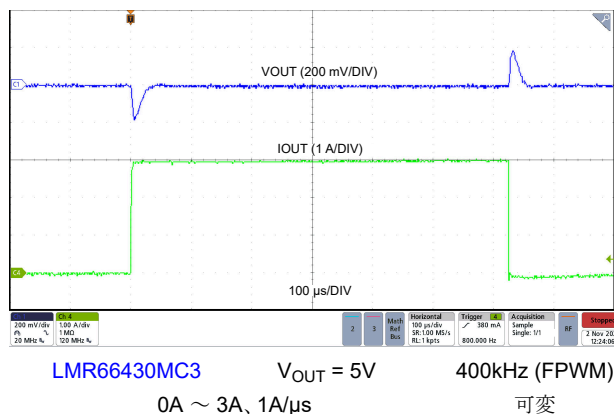
図 8-30. 負荷過渡
