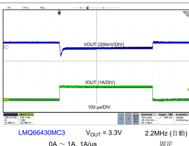
図 8-13. 負荷過渡
