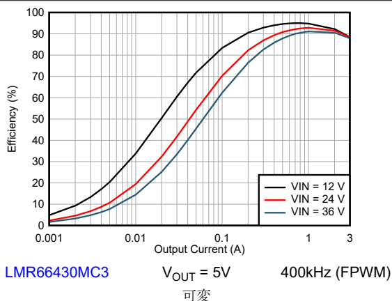
図 8-27. 効率
