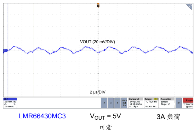
図 8-32. 出力電圧リップル
