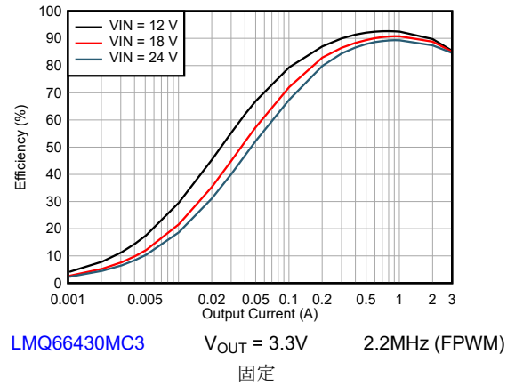
図 8-5. 効率
