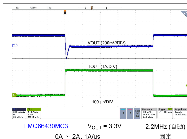
図 8-10. 負荷過渡
