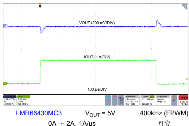
図 8-31. 負荷過渡
