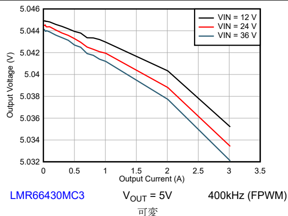
図 8-28. ラインレギュレーションおよびロードレギュレーション
