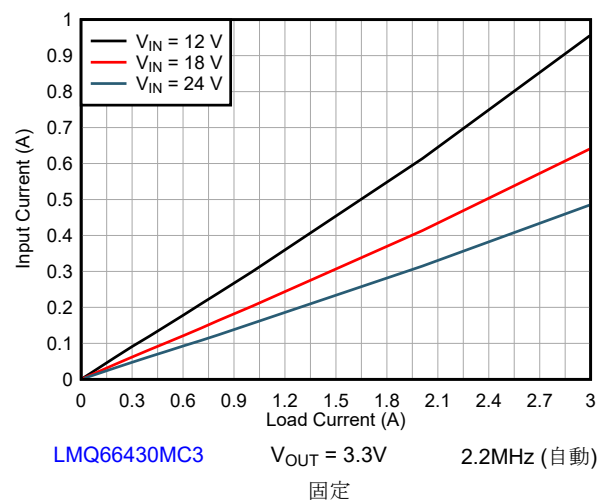
図 8-9. 入力電流と負荷電流との関係
