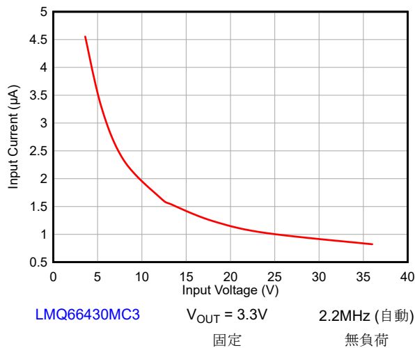
図 8-8. 入力スイッチング電流と入力電圧との関係
