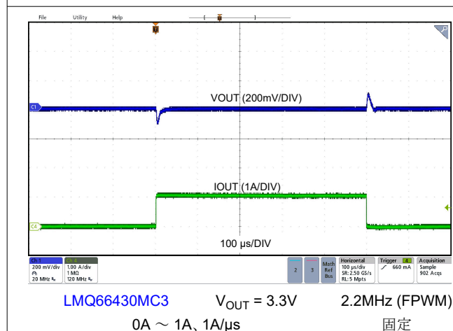
図 8-12. 負荷過渡
