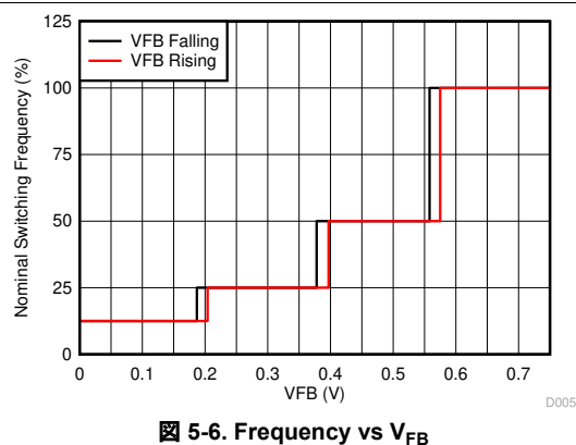
図 5-6. Frequency vs V_{FB}
