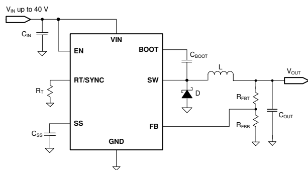
概略回路図
