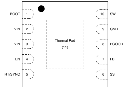
図 4-2. DPR Package 10-Pin (WSO) Top View
