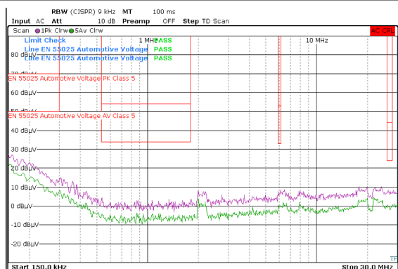
V_{OUT} = 5V F_{SW} = 2MHz I_{OUT} = 1A 周波数スパン: 150kHz ~ 30MHz
