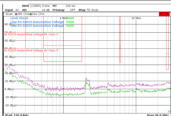
V_{OUT} = 3.3V F_{SW} = 2MHz I_{OUT} = 1A 周波数スパン: 150kHz ~ 30MHz
