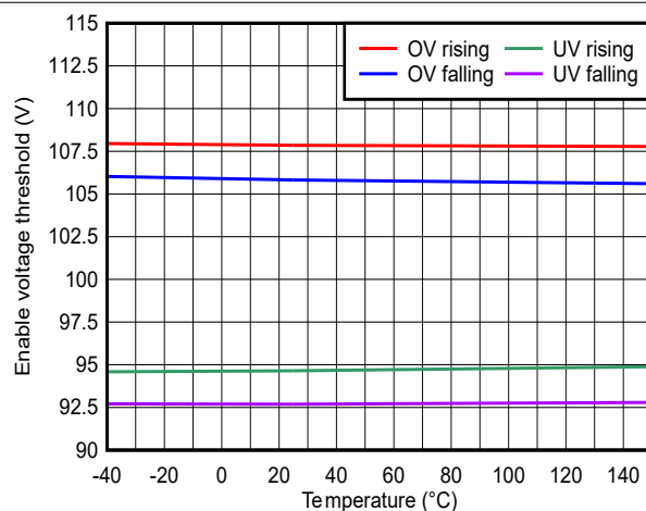
図 6-12. PGGOOD スレッシュホールド
