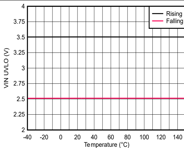
図 6-10. 入力電圧 UVLO - B バリエーション
