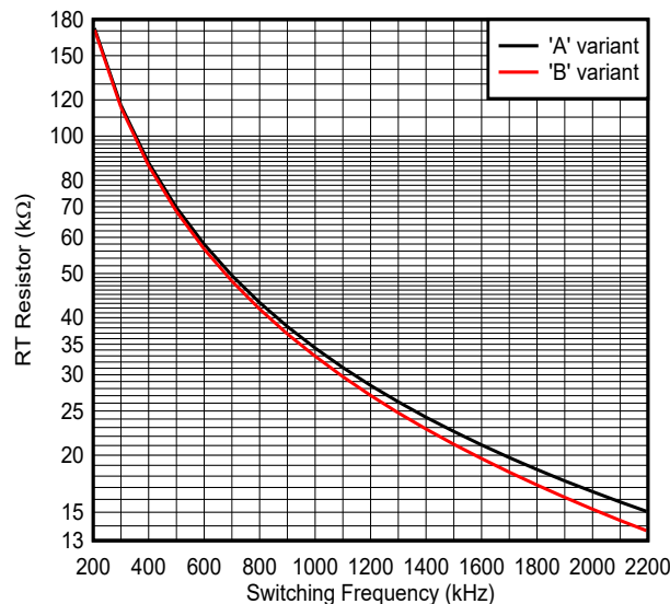
図 7-3. A および B バリエーションの RT 値とスイッチング周波数との関係
