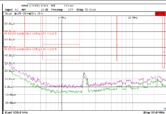
図 8-26. 伝導 EMI と CISPR25 制限値との関係 (紫: ピーク信号、緑: 平均信号)、LMR60440QEV
