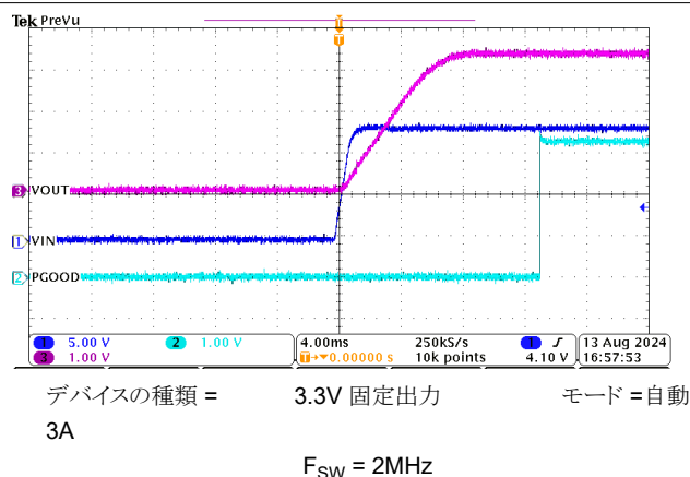
図 8-17. スタートアップ動作
