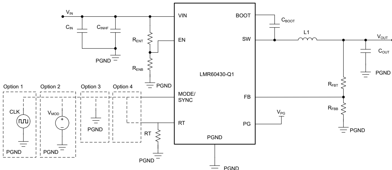
図 8-1. LMR60430-Q1 のリファレンス回路図
