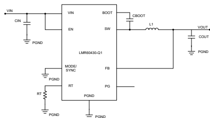
概略回路図 - 固定出力
