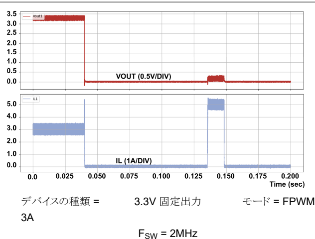
図 8-19. 短絡発生
