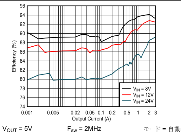
図 8-6. 効率
