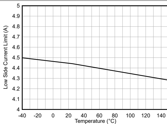
図 6-2. ローサイド MOSFET 電流制限値
