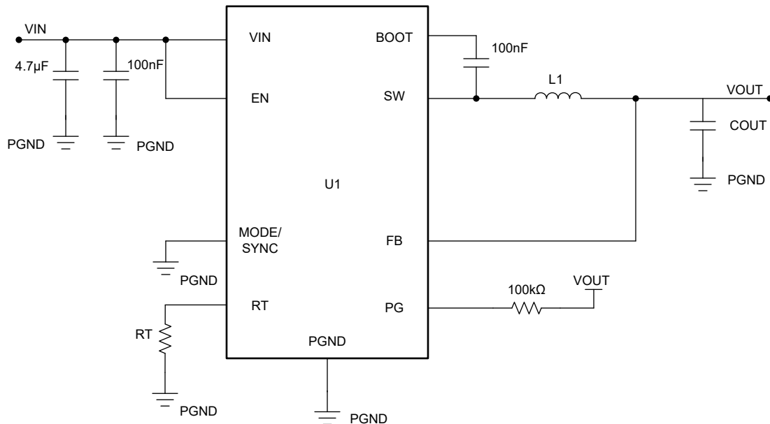
図 8-36. アプリケーション回路例
