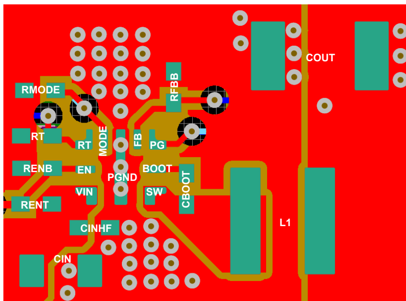
図 8-38. RAK パッケージの推奨レイアウト例 (2.5mm × 2mm)
