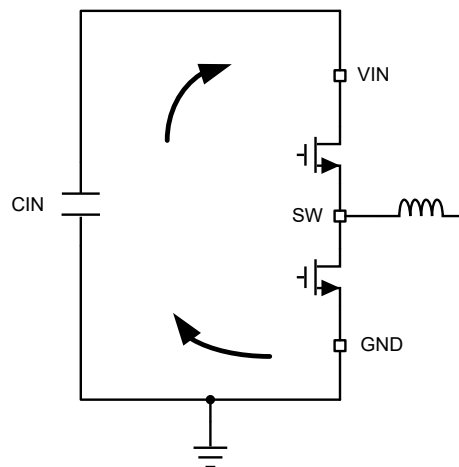
図 8-37. 高速エッジを持つ電流ループ
