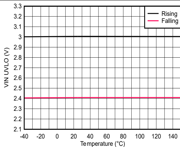
図 6-9. 入力電圧 UVLO - A バリエーション
