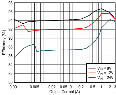
図 8-8. 効率
