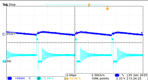
図 8-20. 短絡からの回復
