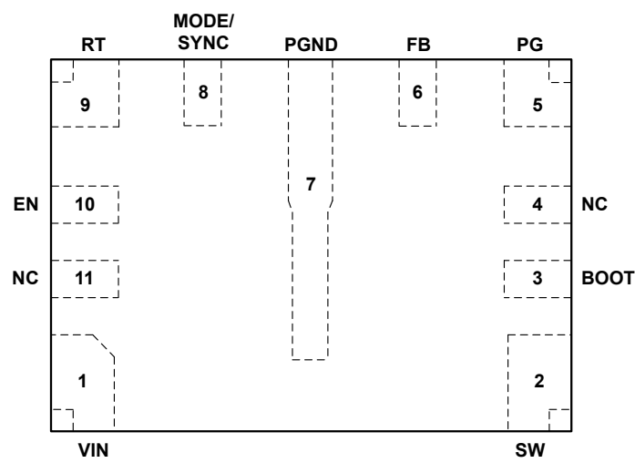
図 5-2. RBM パッケージ 11 ピン WQFN-HR (上面図)
