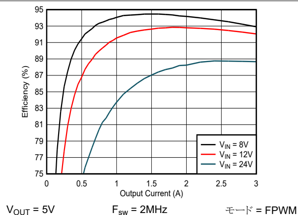
図 8-7. 効率
