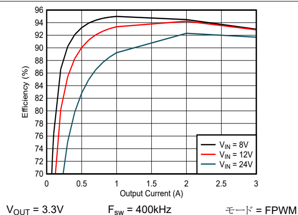
図 8-5. 効率
