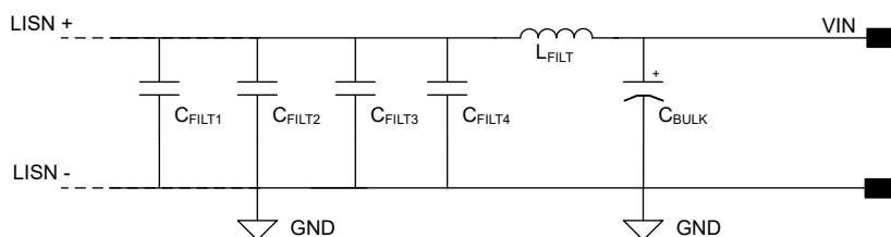
図 8-35. 標準入力 EMI フィルタ回路図
