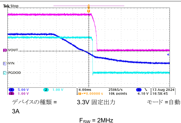
図 8-18. シャットダウン動作
