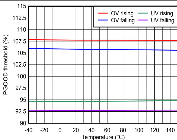
図 6-11. PGOOD スレッシュヨルド
