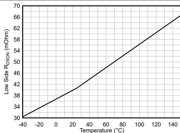
図 6-4. ローサイド MOSFET の R_{DS-ON}
