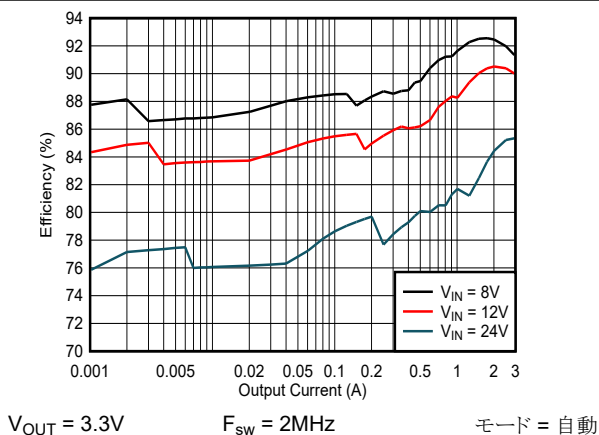
図 8-2. 効率
