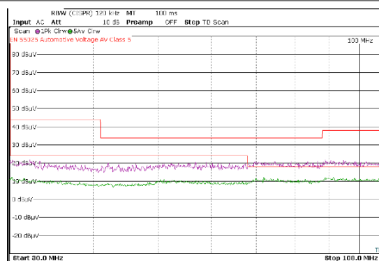
図 8-27. 伝導 EMI と CISPR25 制限値との関係 (紫: ピーク信号、緑: 平均信号)、LMR60440QEV
