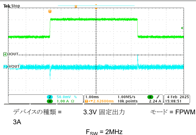
図 8-16. 1.5A ~ 3A の負荷過渡
