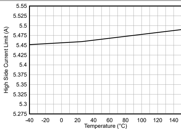
図 6-1. ハイサイド MOSFET 電流制限値
