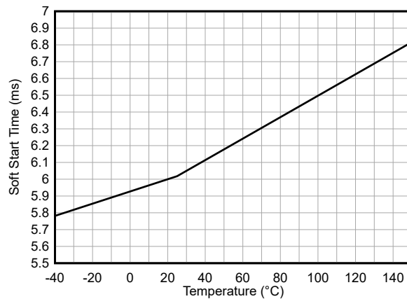
図 6-6. ソフトスタート時間
