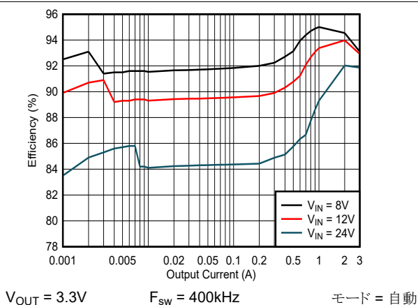
図 8-4. 効率
