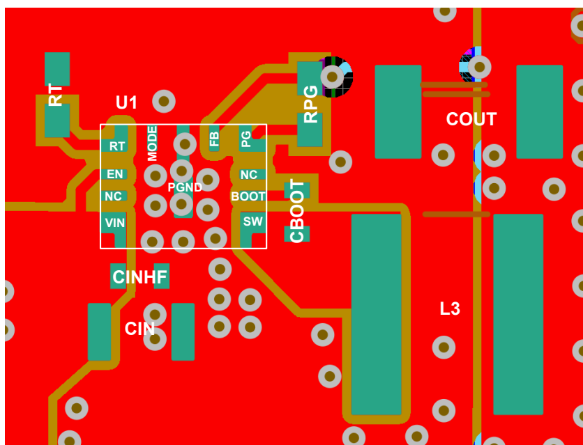
図 8-39. RBM パッケージの推奨レイアウト例 (3.5mm × 2.5mm)
