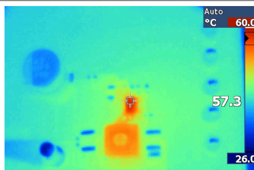
図 8-23. 熱性能
