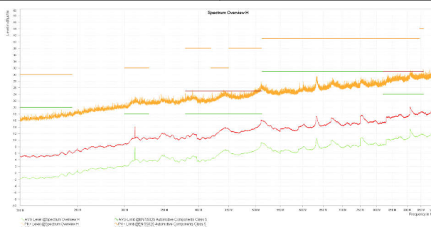
図 8-32. 放射 EMI バイコン水平偏波と CISPR25 制限値との関係、LMR60440QEV
