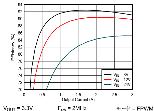
図 8-3. 効率
