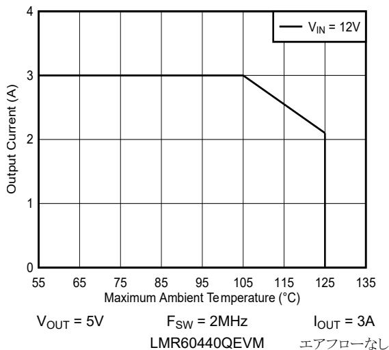
図 8-14. 出力電流と最大周囲温度との関係
