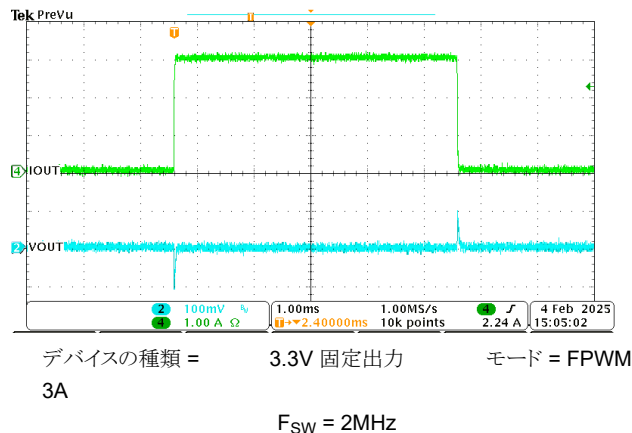
図 8-15. 20mA ~ 3A の負荷過渡
